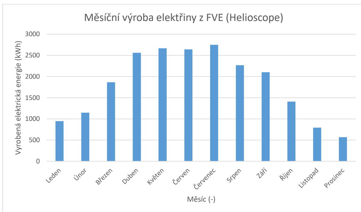
Obrázek 3.4 Grafické znázornění vyrobené elektřiny z FVE v jednotlivých měsících
