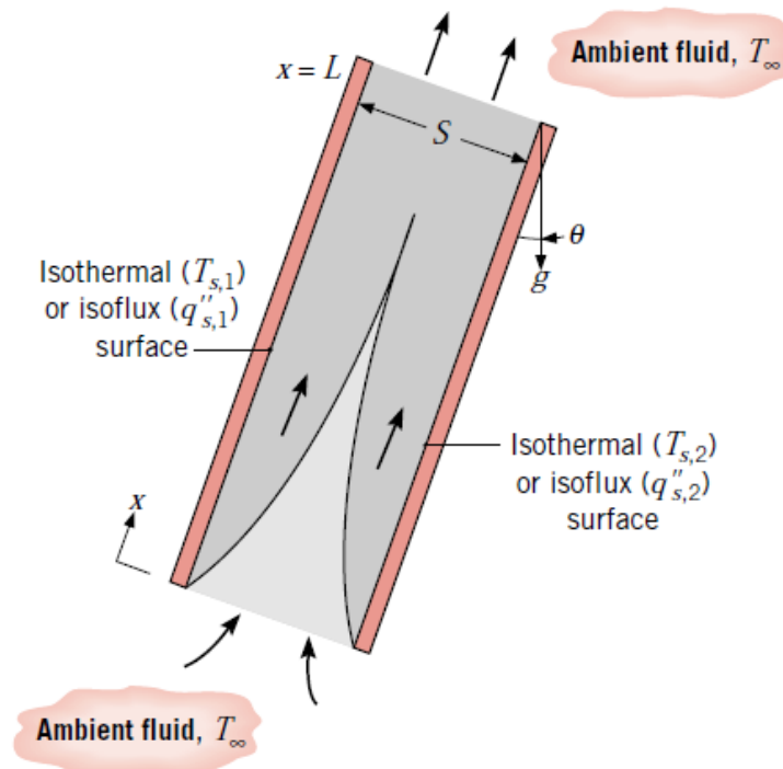
Obrázek 7.4 Proudění přirozenou konvekcí mezi vyhřívánými rovnoběžnými deskami [47]
