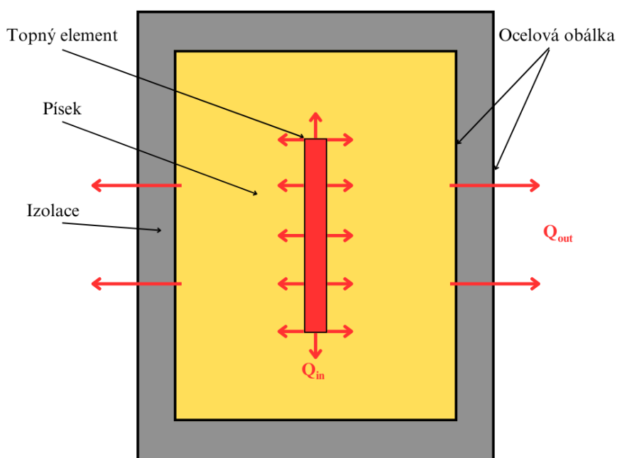
Obrázek 4.2 Koncept pasivně vybíjeného pískového akumulátoru
