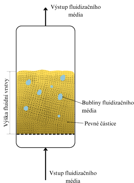
Obrázek 2.4 Základní schéma fluidního lože
