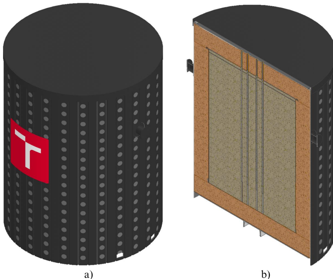
Obrázek 6.1 a) Model Basic b) Podélný řez modelem Basic
