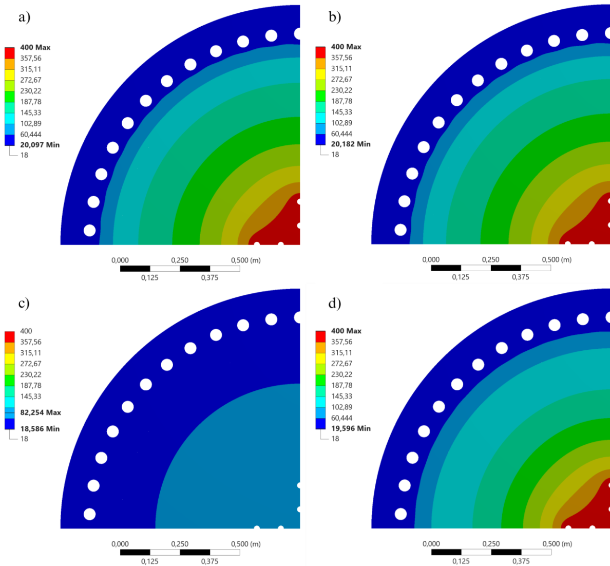
Obrázek 8.13 Teplotní plole v průběhu celoroční simulace modelu s membránovou stěnou a) Červen b) Říjen c) Listopad d) První polovina února
