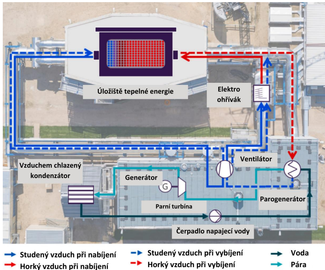
Obrázek 2.15 Schéma zapojení celého zařízení [19]
