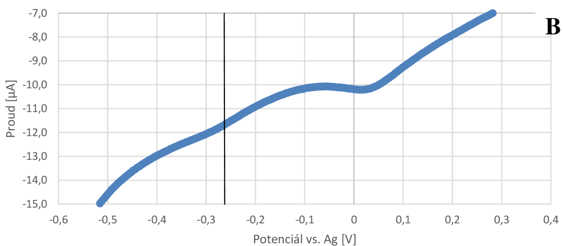
Příloha 2: Transferové adsorpční CSW voltamogramy fentanylu naadsorbovaného ze směrného roztoku fentanylu s heroinem v poměru 1:1000; A – anodický sken, B – katodický sken; frekvence 25 Hz, amplituda 50 mV
