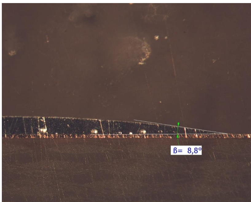
Obrázek 47: Smáčecí úhel pasty 1
