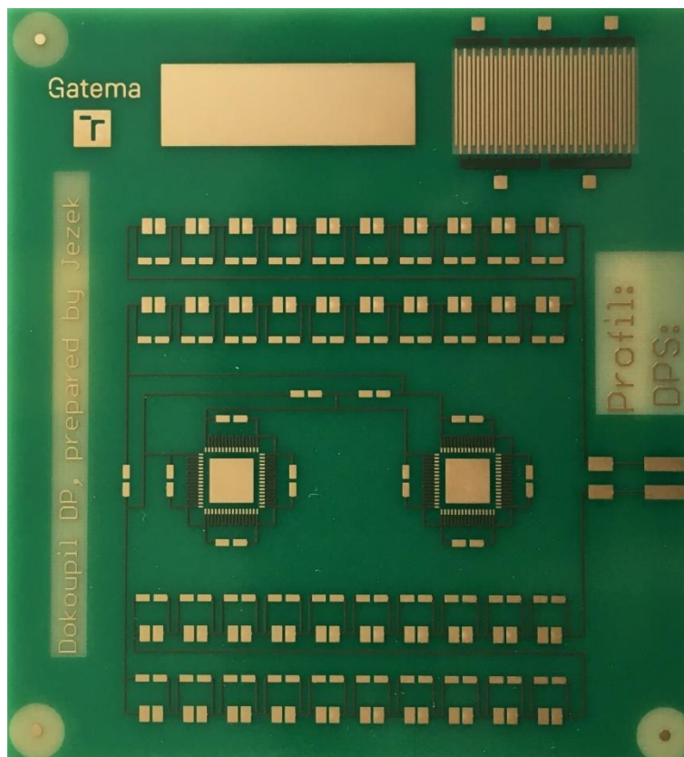
Obrázek 59: Používaná DPS
