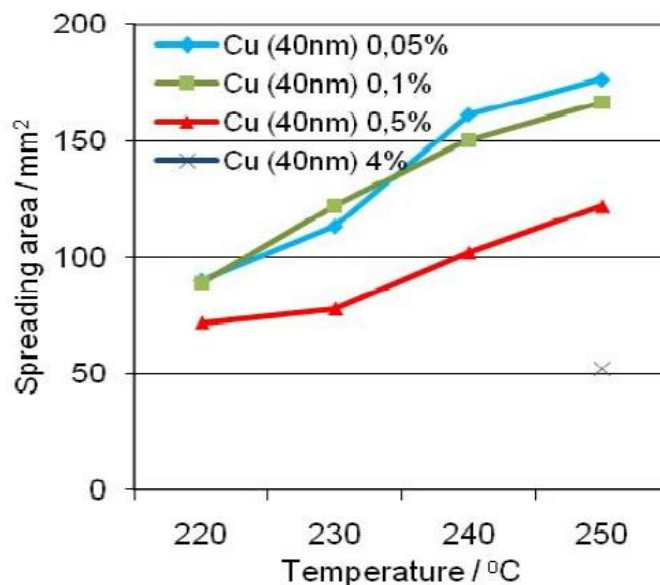
Obrázek 10: Vliv teploty a množství nanočástic na plochu roztékání [5]
