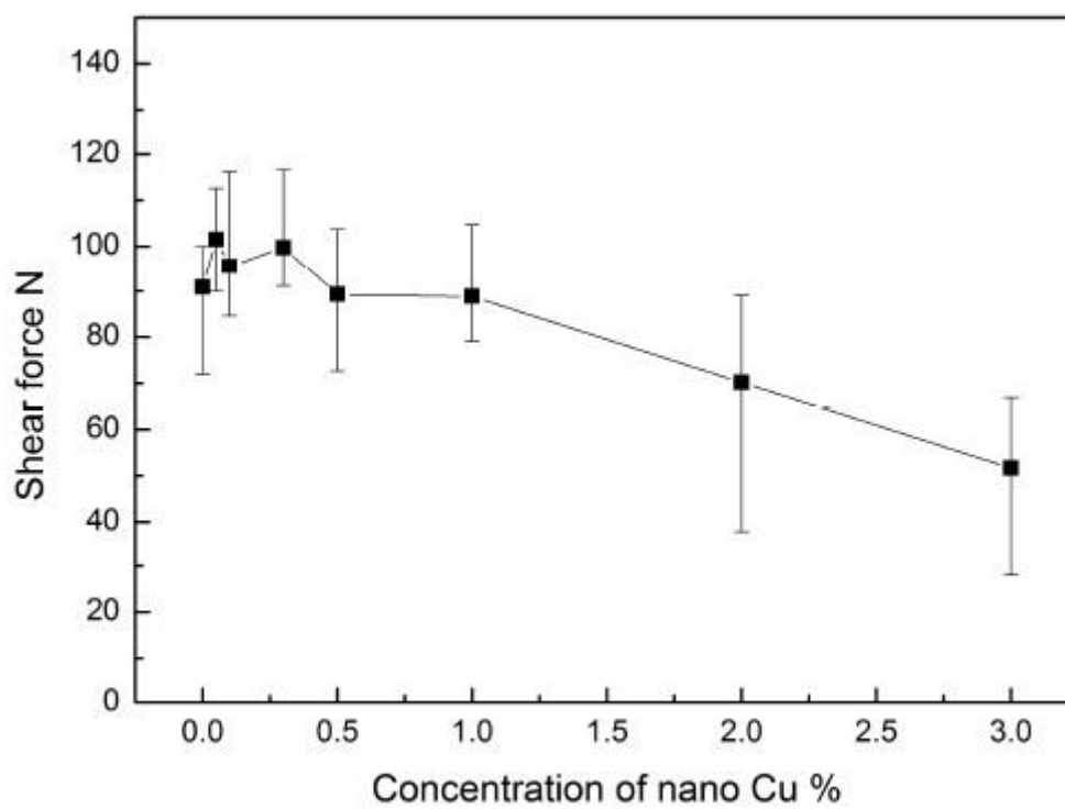
Obrázek 8: Velikost střížné síly v závislosti na počtu nanočástic [4]
