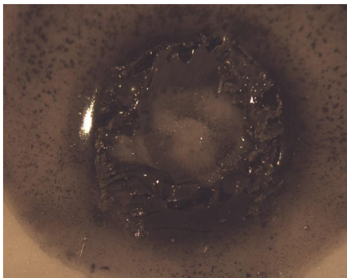
Obrázek 39: Zbytky pasty po neúplném přetavením pasty 4
