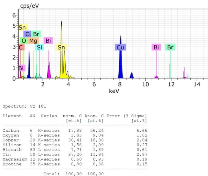
Obrázek 58: Prvková analýza IMC mikrovýbrusu pasty 2
