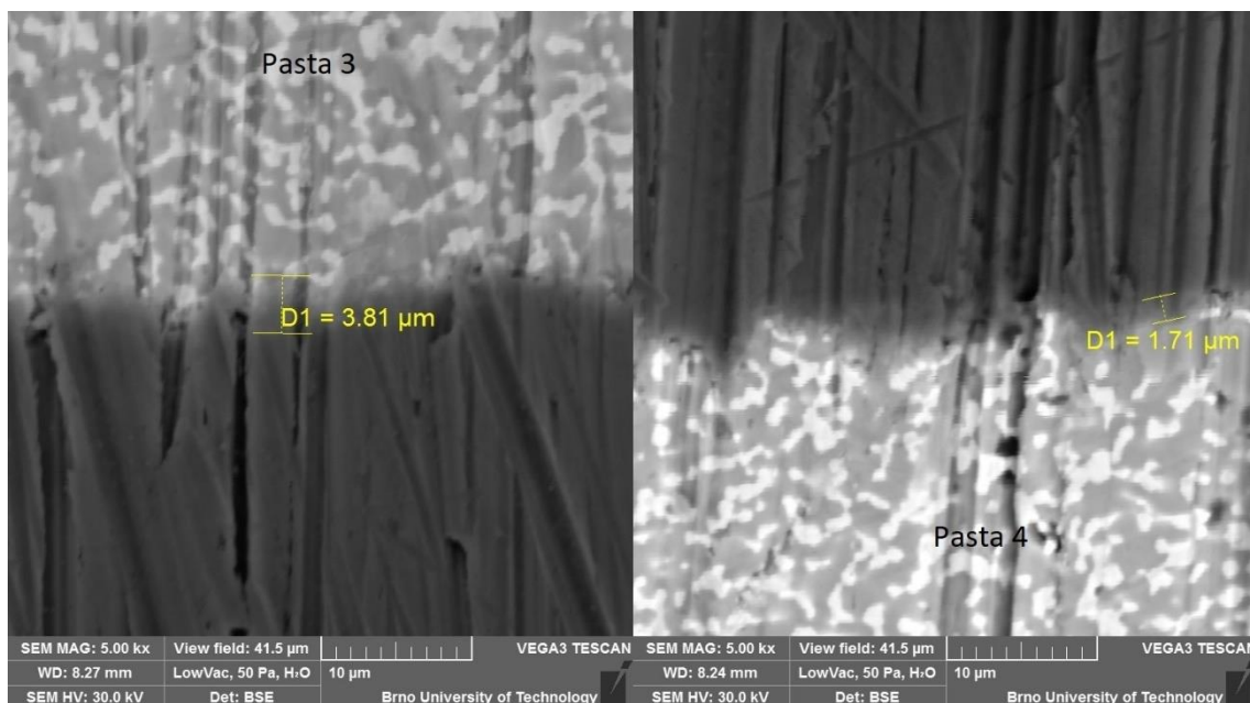
Obrázek 57: Tloušťka IMC pasty 3 a 4
