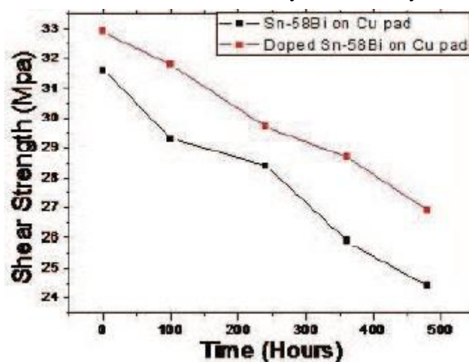
Obrázek 11: Rozdíl maximální síly sříhu mezi obyčejnou Sn-Bi pastou a Sn-Bi pastou s 2 %wt Ag [6]
