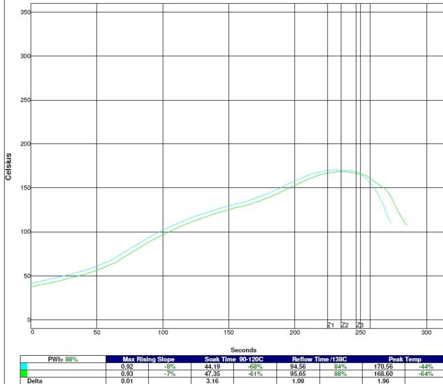
Obrázek 29: Teplotní profil na keramické desce
