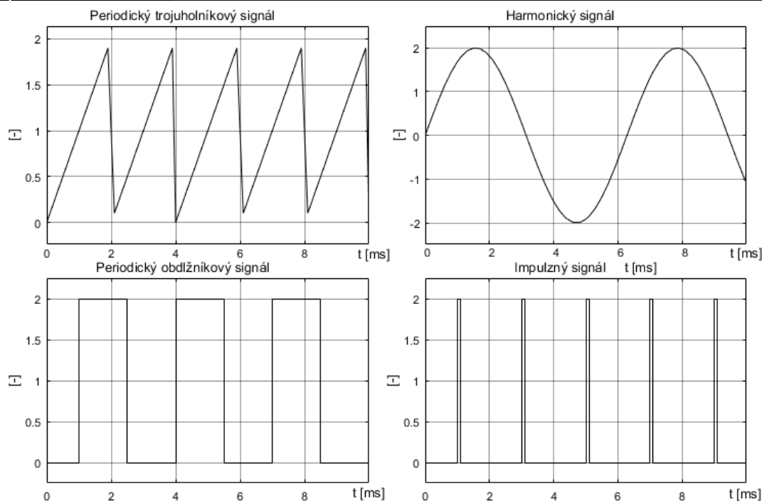
Obr. 2.1.1 – Základné tvary generovaných signálov
