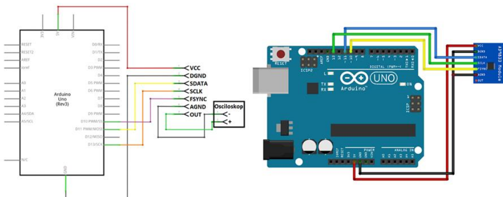
Obr. 3.3.2 – Pripojenie modulu s Arduino [8]
