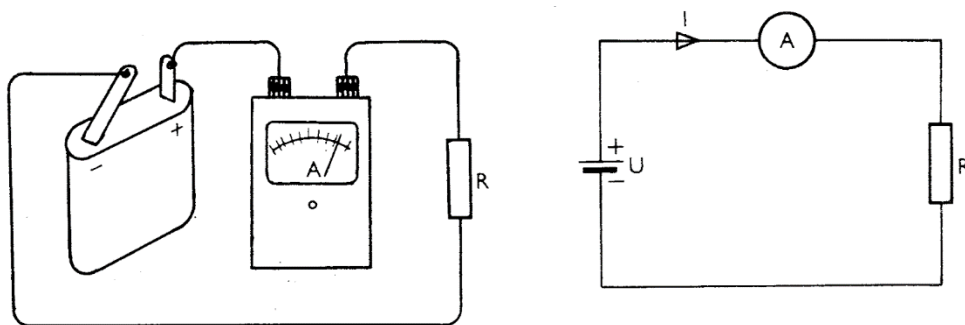
Obr. 7.1. Schéma zapojenia merania [18]
