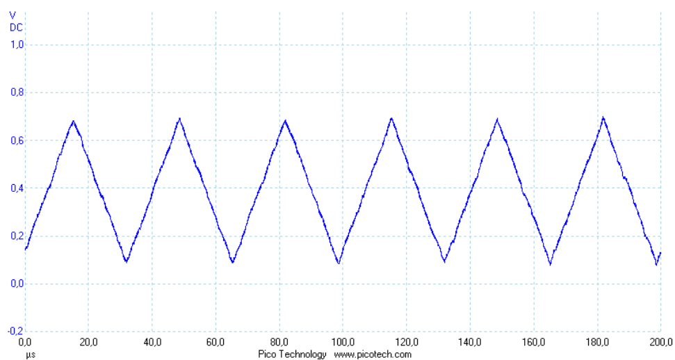
Obr. 6.2.3 Trojuhelník 30kHz
