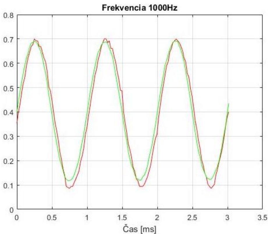
Obr. 6.4.4 Porovnanie signálov sínus 1000Hz
