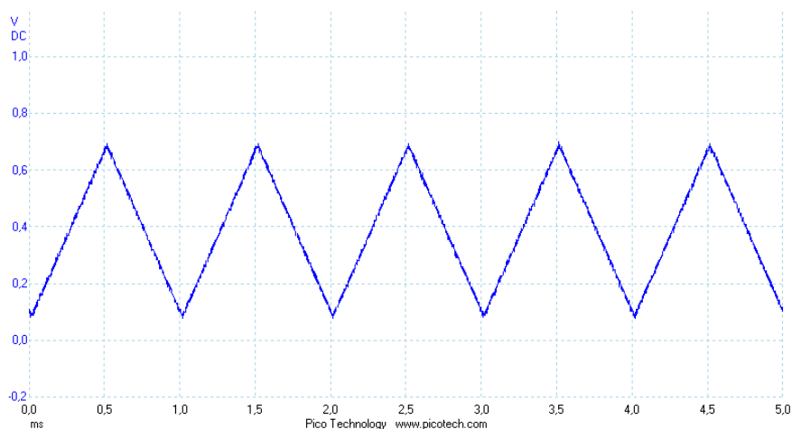
Obr. 6.2.1 Trojuhelník 1000Hz
