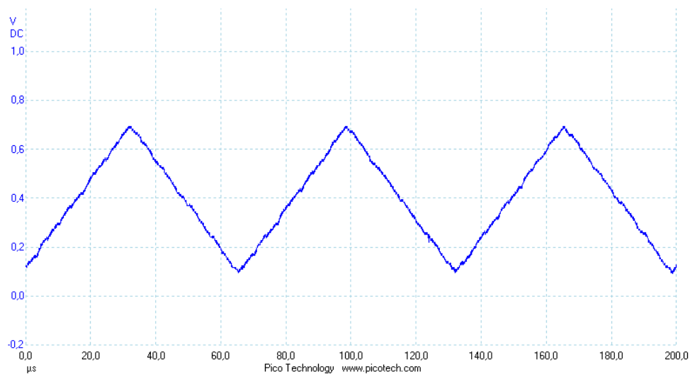
Obr. 6.2.2 Trojuhelník 15kHz
