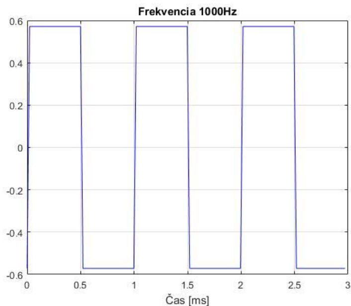
Obr. 6.4.3 Obdĺžnik 1000Hz
