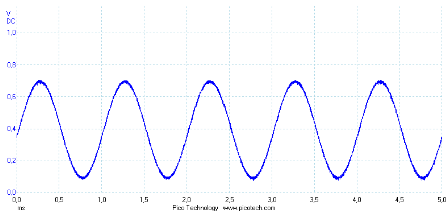
Obr. 6.1.1 Sínus 1000Hz
