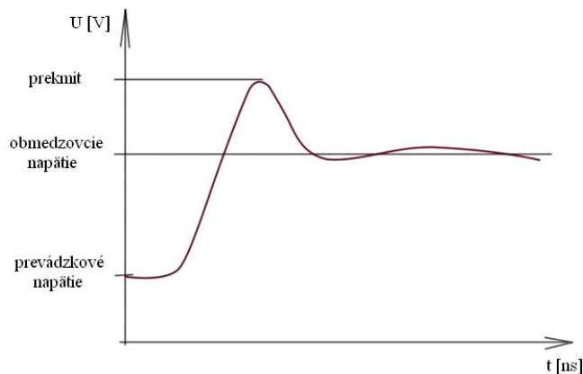
Obr. 7-4 Priebeh napätia pri rýchlej zmene prúdu vo varistore [14].
