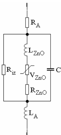
Obr. 7-3 Náhradná schéma varistora ZnO [14].
