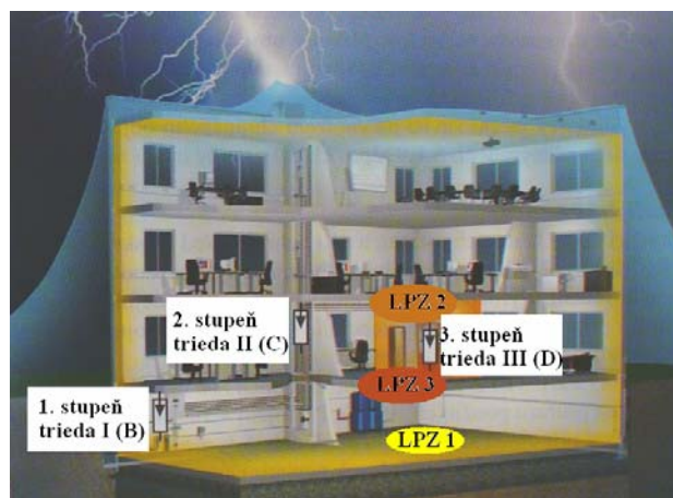
Obr. 5-2 Rozmiestnenie SPD na rozhraní LPZ [5].
