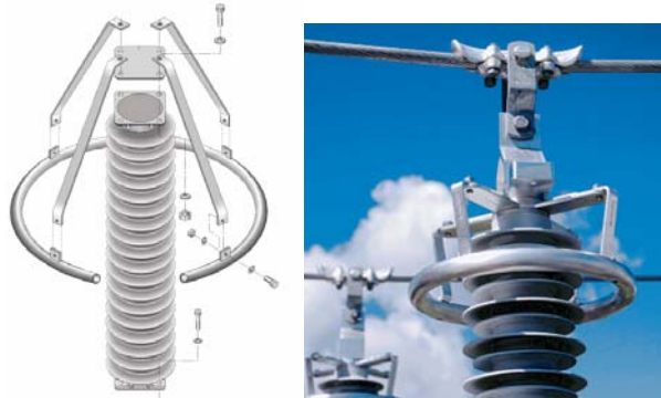
Obr. 7-10 Ochranný kruh zvodíča ZnO [2].
