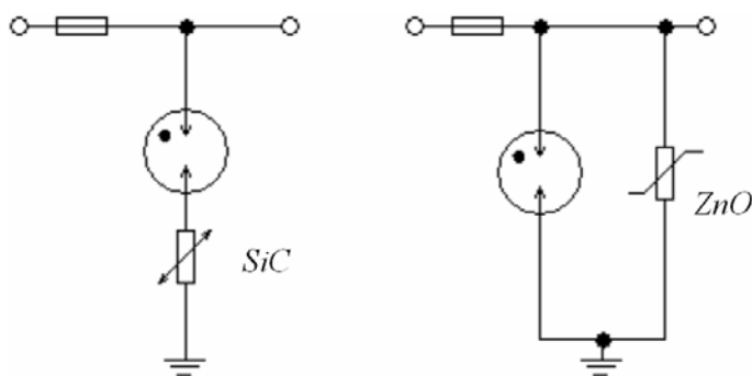
Obr. 7-5 Zapojenia plynom plnených bleskoistiek alebo iskrísk s varistorami.
