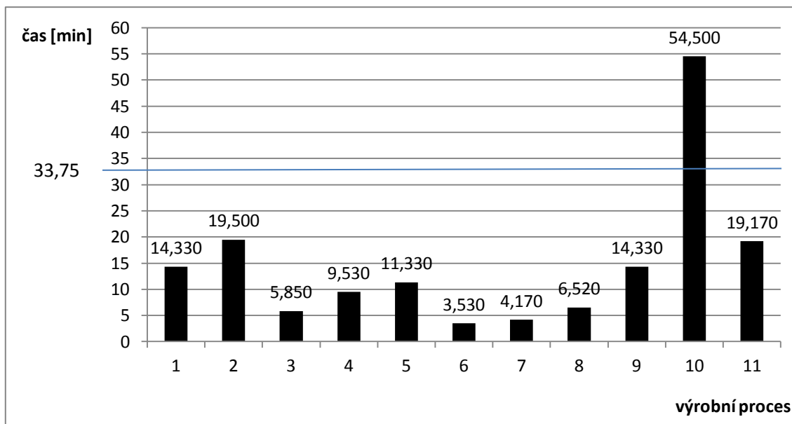
Graf 3: Srovnání cyklových časů s časem taktu (Zdroj: vlastní zpracování)
