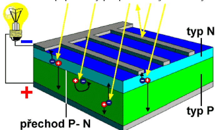
Obrázek 2: P-N přechod [7].
