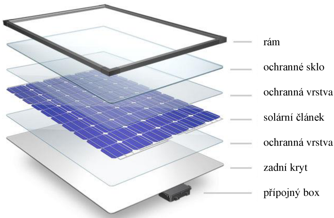
Obrázek 3: Průřez panelem [8].
