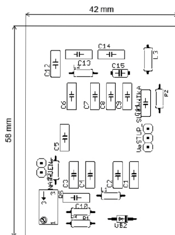
Obr. 0.3 Osazená deska obvodu TDA7088T
