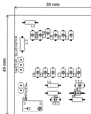
Obr. 0.2 Osazená deska obvodu TDA7021T
