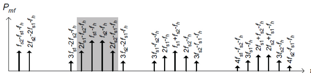
Obr. 1.10 Intermodulační produkty [3]
