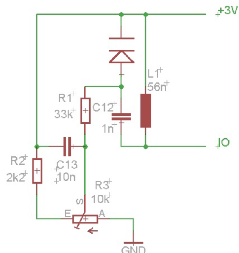
Obr. 2.6 Přelaďování obvodu TDA7021T
