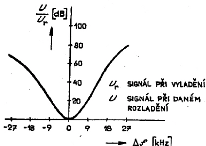
Obr. 1.9 Křivka jednosignálové selektivity přijímače [1]
