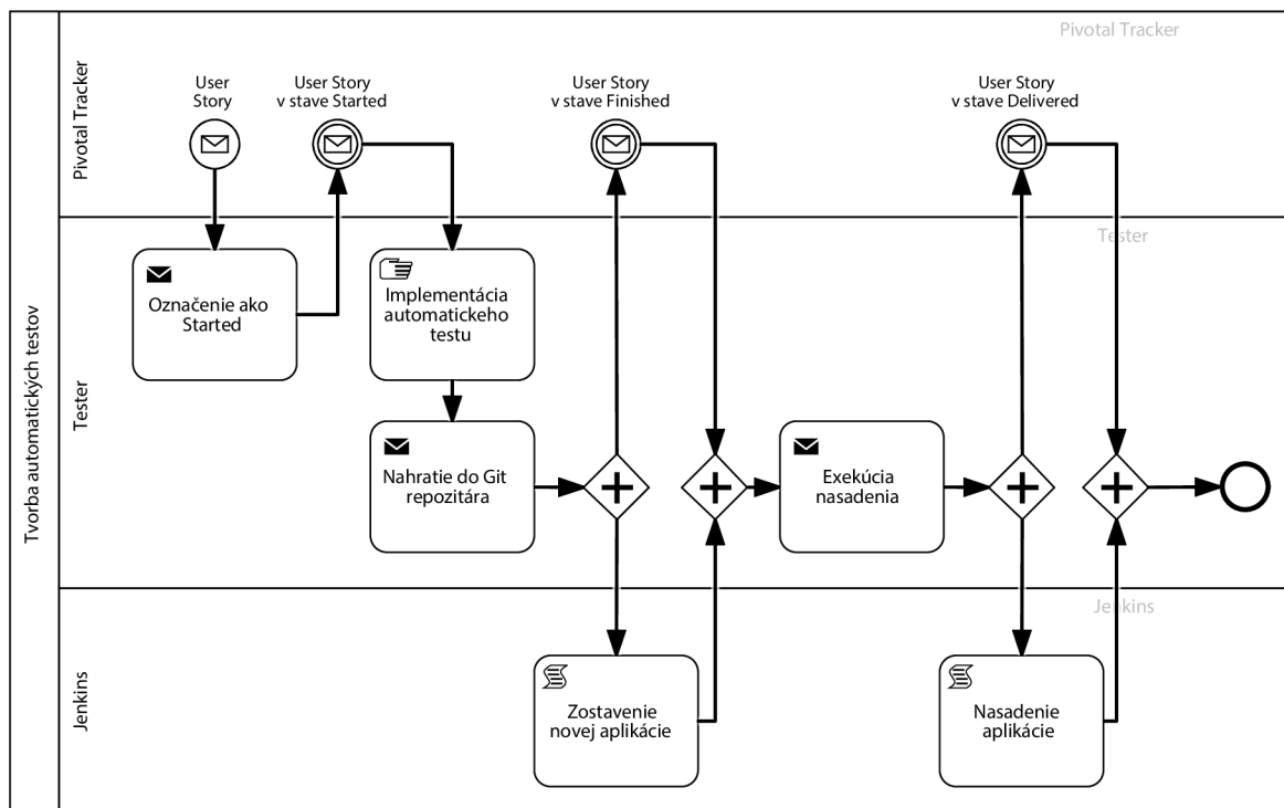
Obr. 5.5: BPM - Tvorba automatických testov (vlastné spracovanie)
