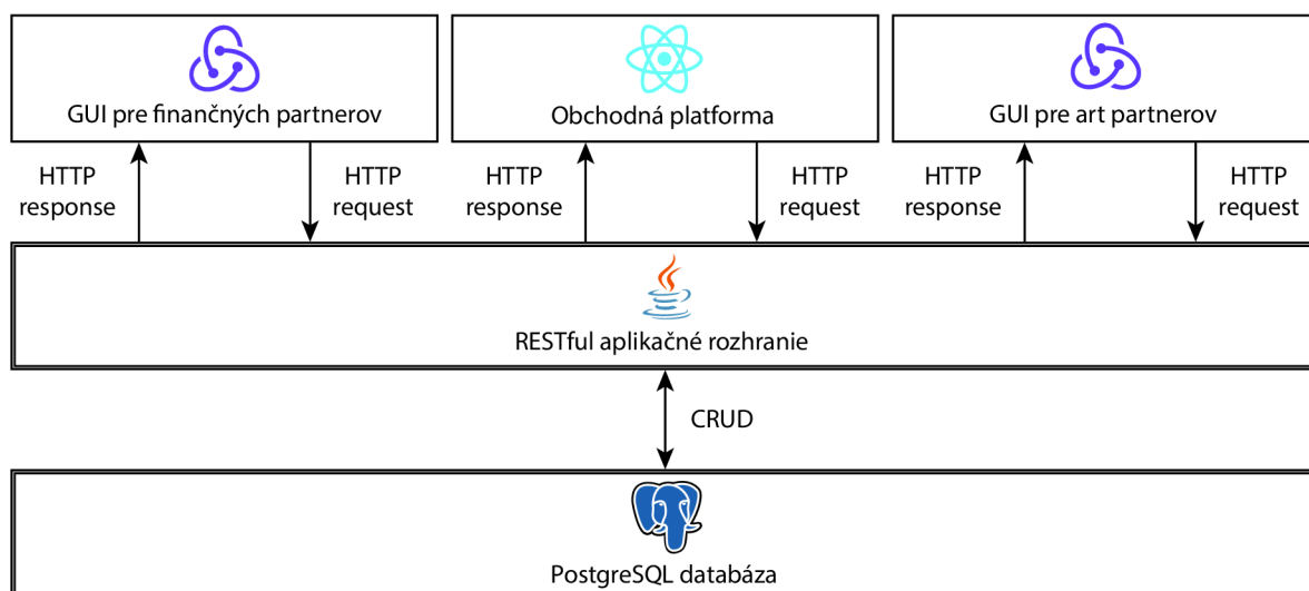
Obr. 4.2: Architektúra systému Artstaq (vlastné spracovanie)
