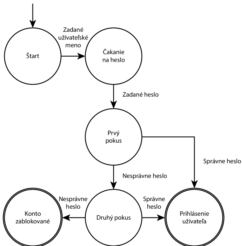
Obr. 3.4: Príklad prihlasovania skrz stavové prechody (vlastné spracovanie)
