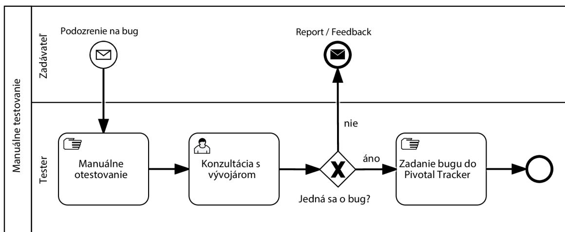
Obr. 5.8: BPM - Manuálne testovanie (vlastné spracovanie)
