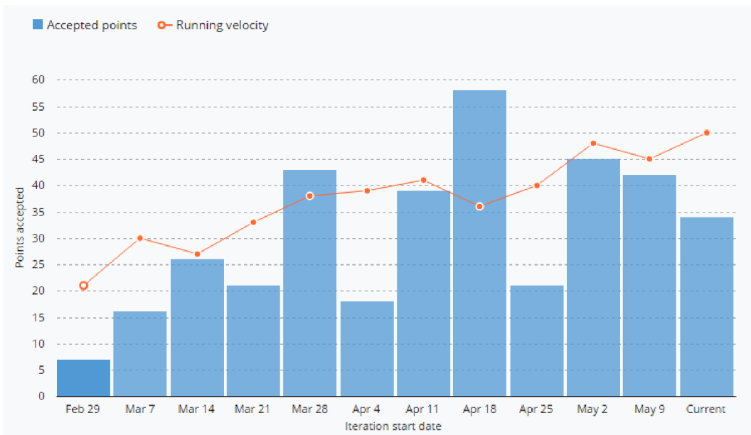
Obr. 6.3: Vykonané testy [42]
