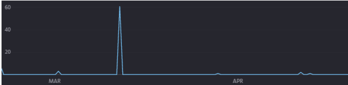
Obr. 6.2: Závažné defekty [43]
