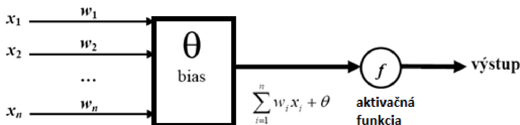
Obrázok 3.1 Perceptrón (prepracované z [1])
