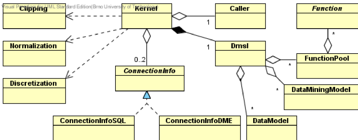
Obrázok 4.2 Diagram základných tried jadra (prevzaté z [9])
