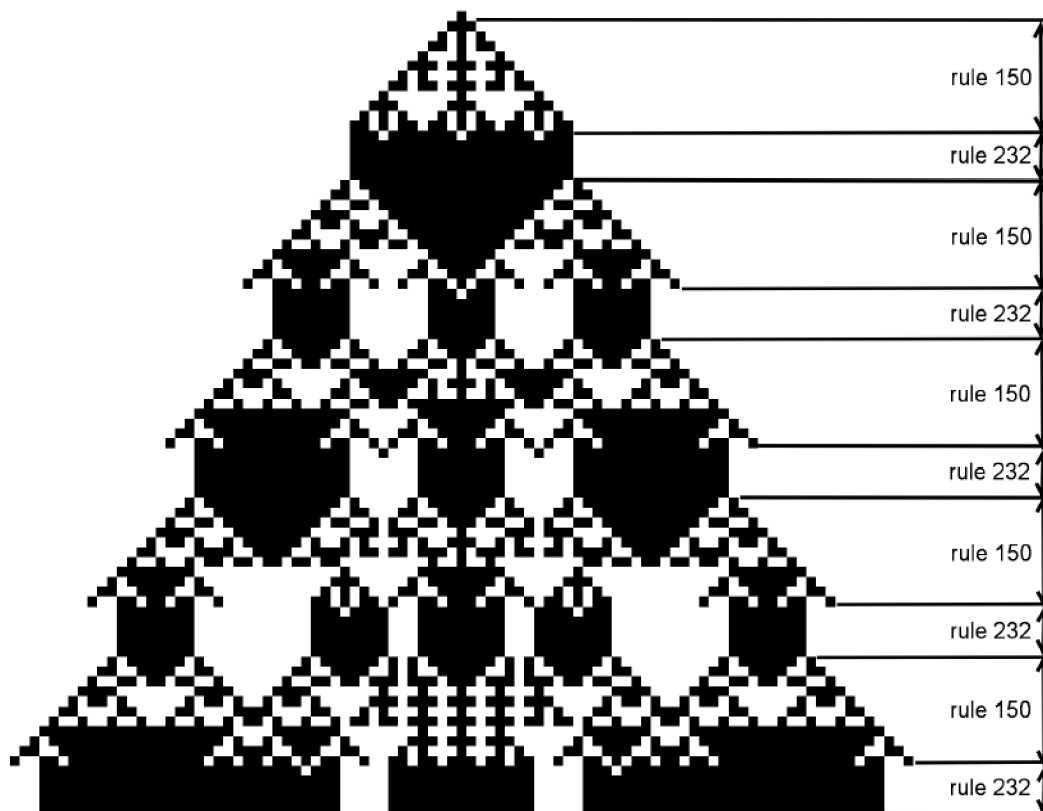
Obrázek 4.1: Ukázka vývoje 1D CA s globálním řízením [13]
