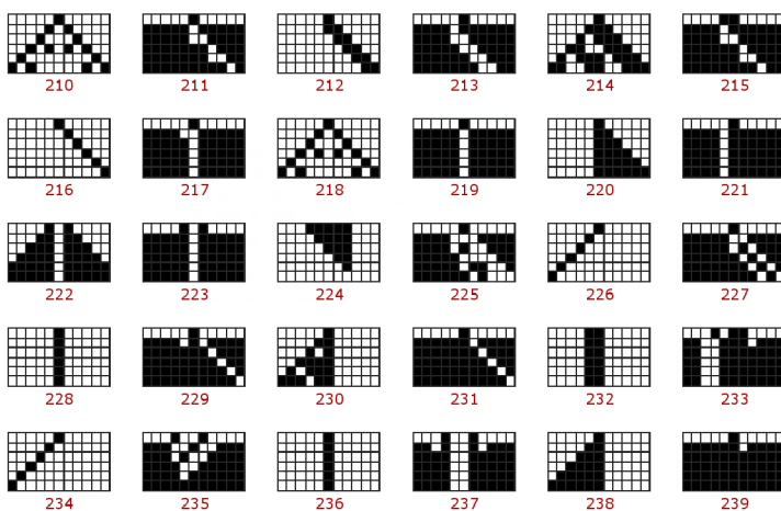
Obrázek 3.10: Pravidla 210 - 239 [22].
