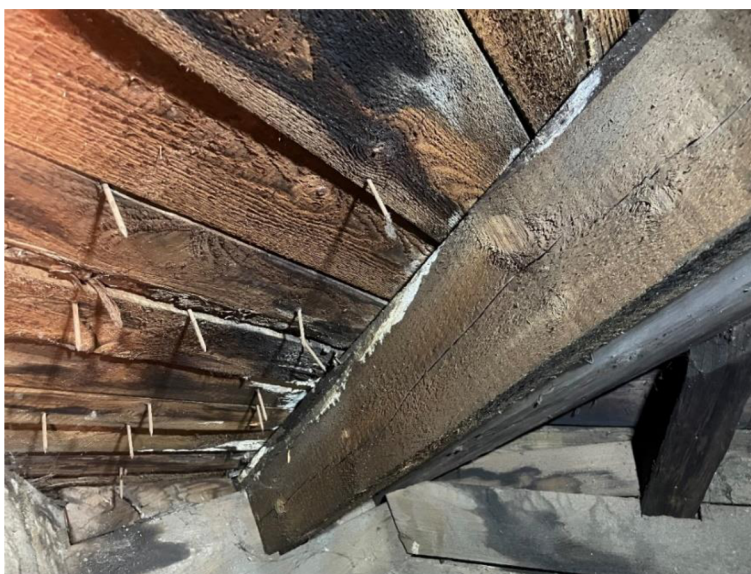
Obrázek 5.1.1.2: Šíření plísní na spodní ploše bednění jihovýchodního námětku z důvodu zatékání.
