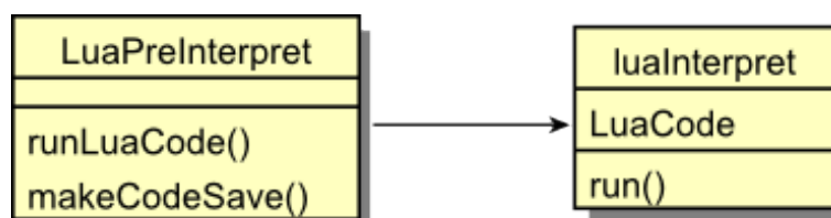
Obrázek 5.3: Třídy části interpretu LUA
