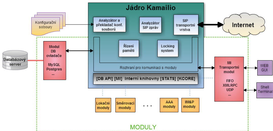
Obr. 2.2: Architektura Kamailio
