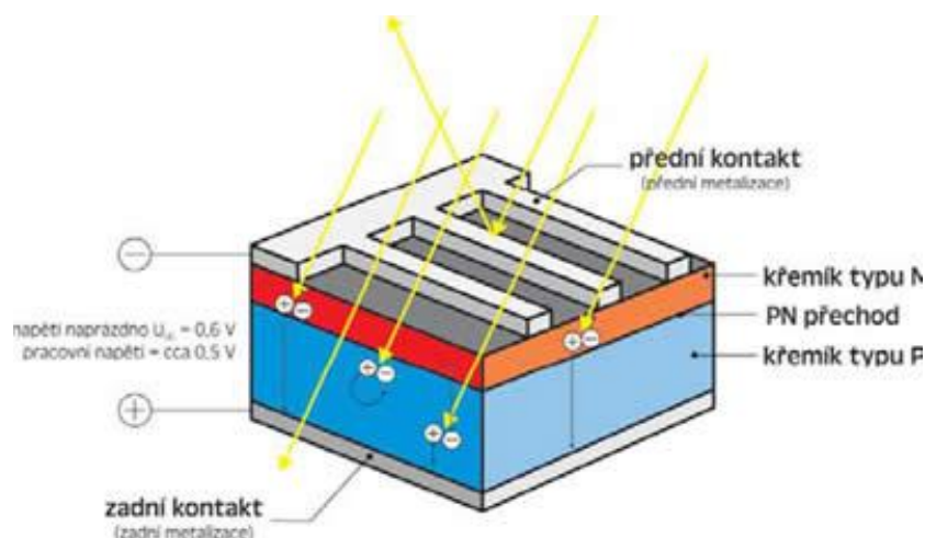
Obr. 2-5 Princip činnosti solárního článku [3]
