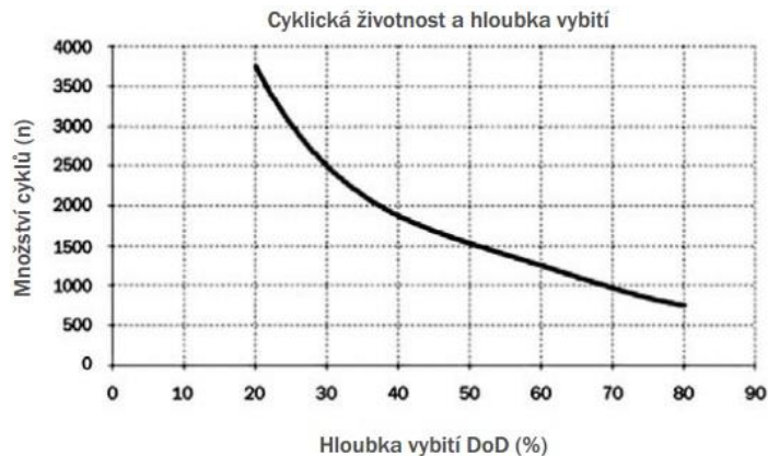
Obr. 2-10 Závislost počtu cyklů na procentuálním vybití akumulátoru [16]
