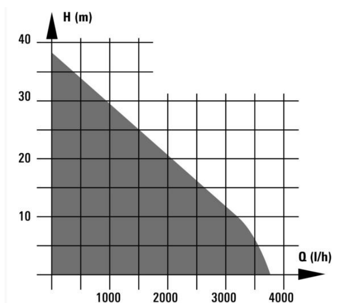
Obr. 1-3 Charakteristika čerpadla [13]
