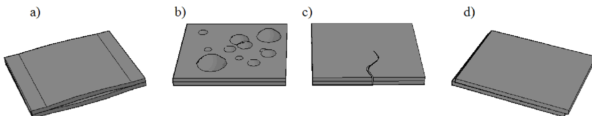
Obr. 11 : a) Delaminace LTCC pásků, b) bubliny, c) vertikální praskliny, d) vzájemné posunutí vrstev
