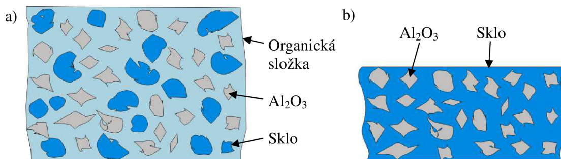
Obr. 2 : Funkce skla ve struktuře LTCC a) před výpalem b) po výpalu
