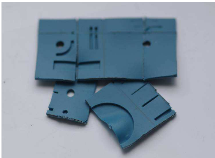
Obr. 28 : Výpalem zdeformovaná struktura vytvořená LTCC keramikou DuPont 951
