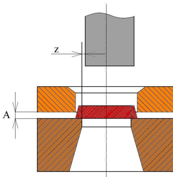
Obr. 12 Schéma přistříhovacího nástroje [13]
