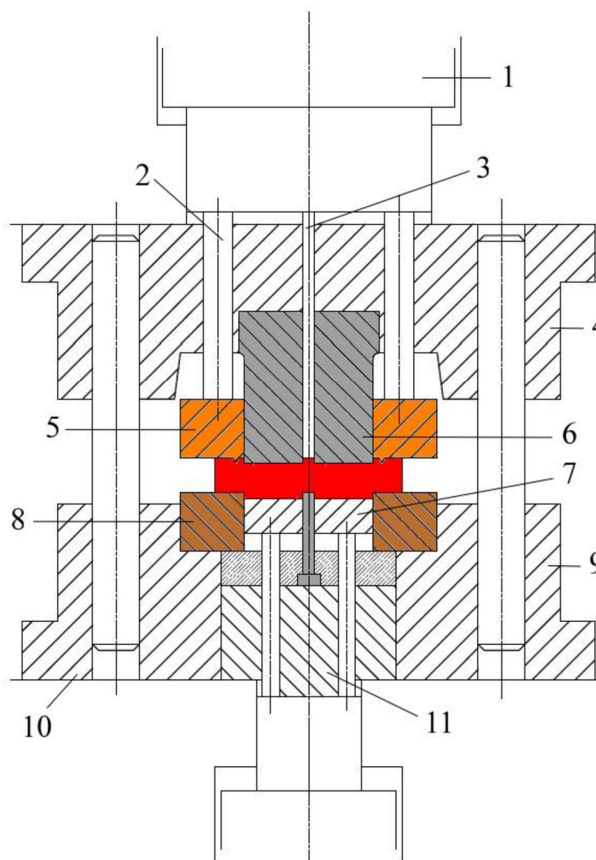
Obr. 9 Schéma nástroje s pevným střížníkem a pohyblivým přidržovačem [7]
