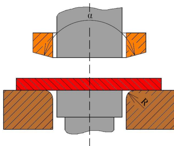
Obr. 6 Stříhání se zkoseným přidržovačem [13]
