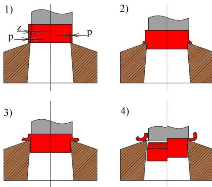
Obr. 8 Postup při přistříhování [7]
