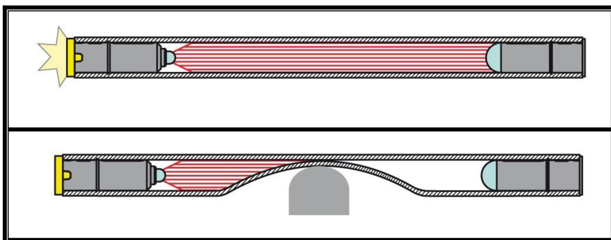
Obr. 35) Princip nárazníku a lišty s optoelektronickým senzorem [53]
