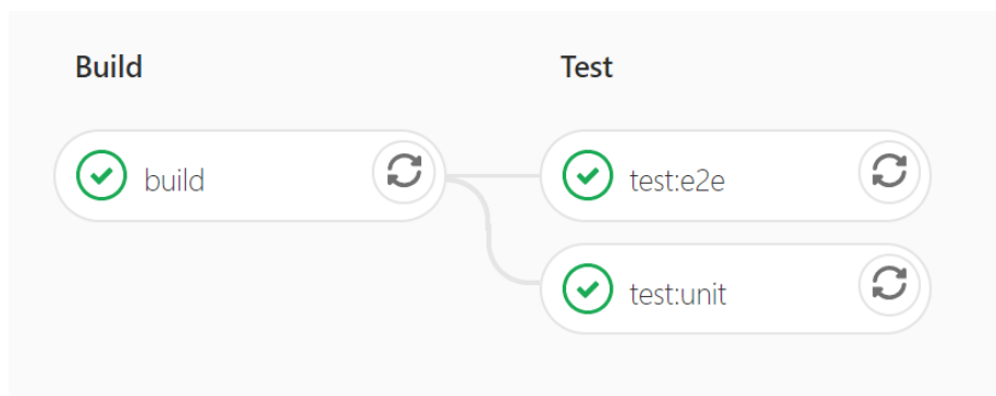
Obrázek 6.2: Etapy GitLab CI/CD jsou rozděleny do fází. Fáze probíhají sekvenčně a pokud jedna neuspěje, následující jsou přeskočeny. (zdroj: autor)
