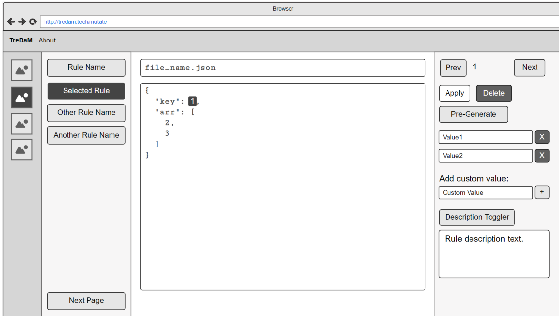
Obrázek 4.3: Návrh stránky pro aplikování mutačních pravidel. Seznam pravidel levého panelu nahradil ovládací prvky předchozí stránky. Pravý panel obsahuje popis zvoleného pravidla a přidány jsou další ovládací prvky s činností spojené. Následující stránky respektují rozložení informací a rozhraní je tak konzistentní. (zdroj: autor)
