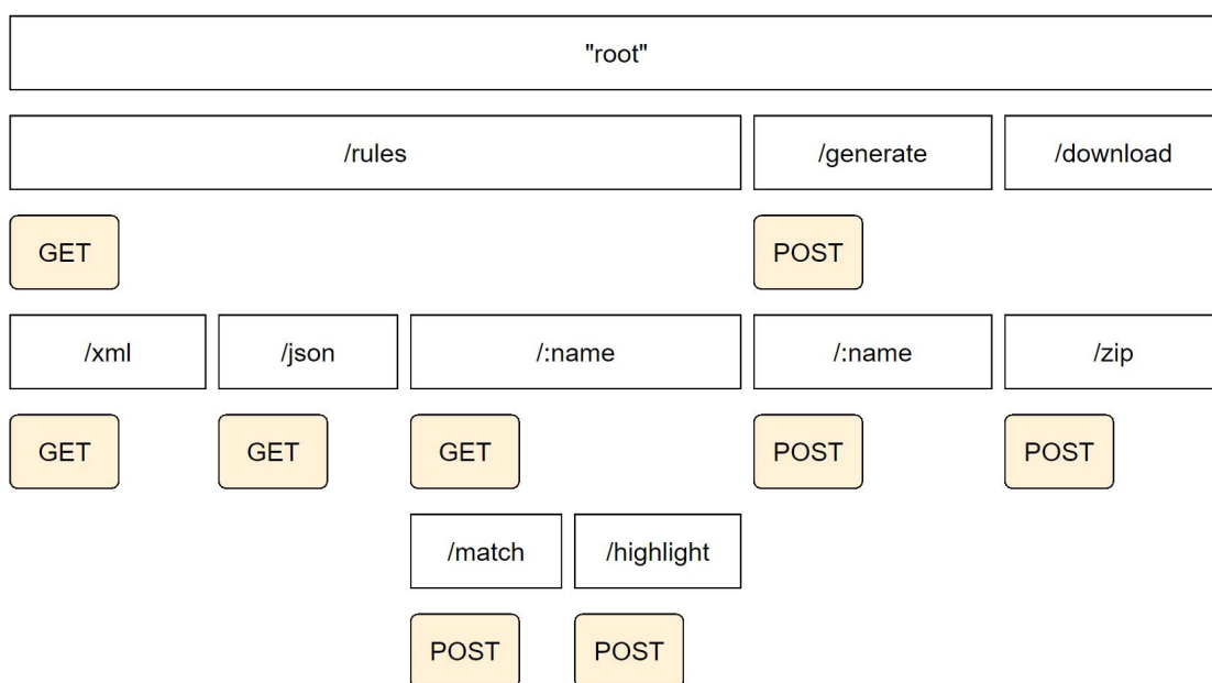
Obrázek 4.5: Grafické znázornění koncových bodů REST rozhraní serveru. Každý koncový bod je definován adresou URL a metodou HTTP. Slouží pro poskytování dat a funkcionalit pro klientskou aplikaci. (zdroj: autor)
