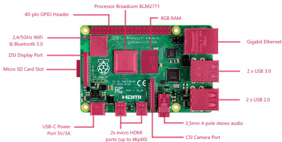
Obrázek 4.5: Počítač Raspberry Pi model 4B (zdroj: [54])
