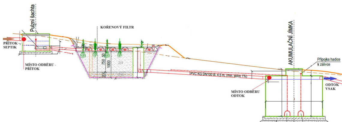
Obr. 14: Místa odběrů odpadní vody na KČOV, převzato a upraveno ze stavební dokumentace Ing. Libor Teplý (2019)
