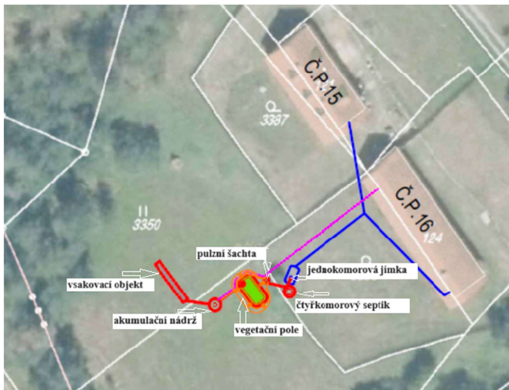
Obr. 10: Situační zobrazení KČOV Žďár 15, převzato z projektové dokumentace Ing. Libor Teplý
