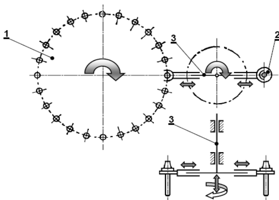
Obr. 12. Systémy AVN s výměnou zásobník-manipulátor-vřeten [2]
