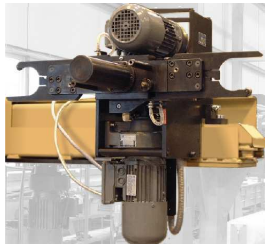
Obr. 26 - Manipulátor fy. TOS VARNSDORF [5]
