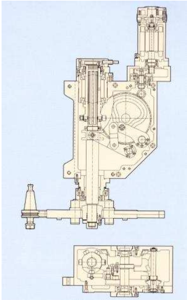
Obr.27 - Manipulátor [13]
