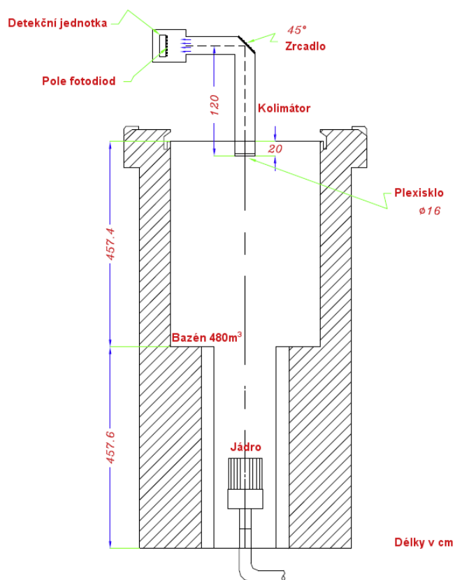
Obr. 3-3: Nákres reaktoru s uspořádáním experimentu [20]
