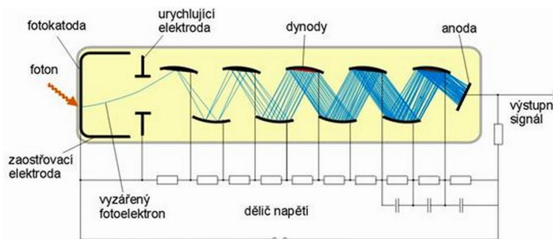
Obr. 4-2: Princip fotonásobiče [11]
