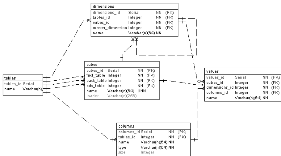
Obrázek 8.1: Fyzické ERD schéma uložení a provázání metadat
