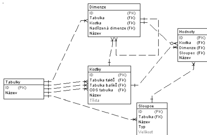
Obrázek 6.1: Logické ERD schéma uložení a provázání metadat
