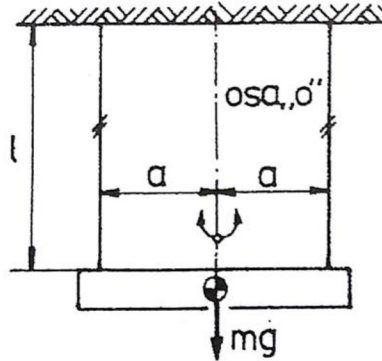
Obr. 26 bifilární závěs [5]
