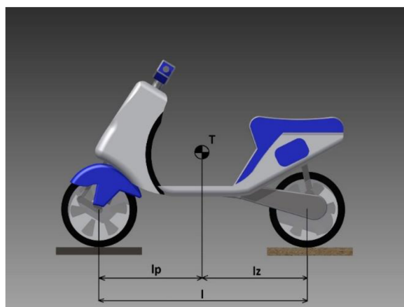
Obr. 15 Hledané rozměry pro určení polohy těžiště v podélném směru
