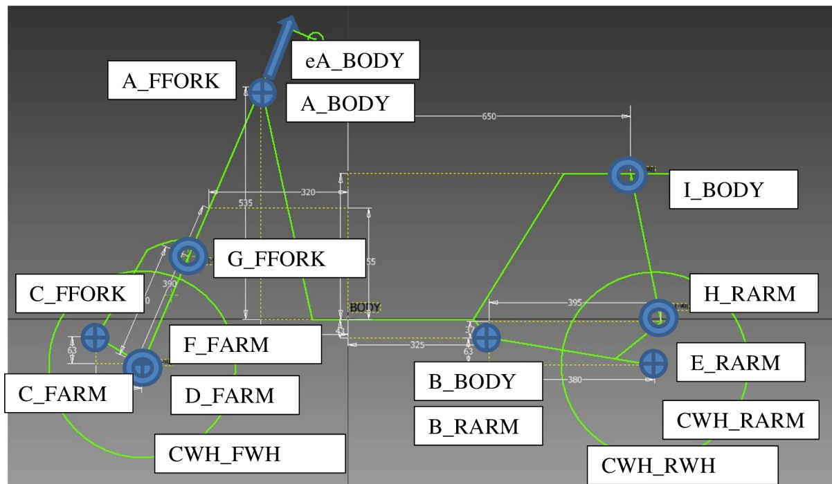
Obr. 13 Kinematický model motocyklu Piaggio Zip SP
