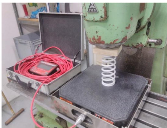
Obr. 38 Metodika měření tuhosti pružiny
