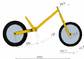
Obr. 3 Důležité body a vzdálenosti modelu EMEA040 [2]
