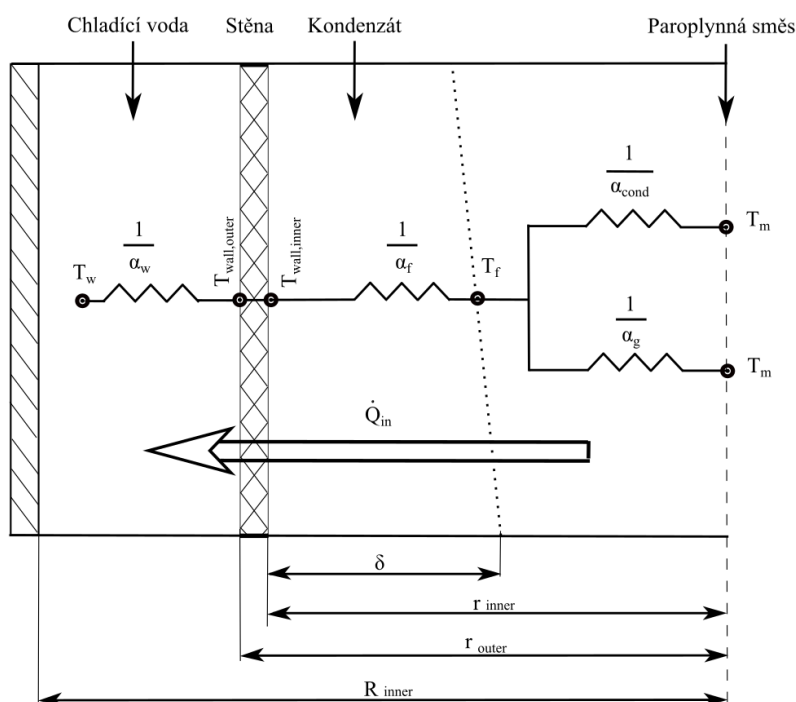
Obr. 2 Přestup tepla z proudu parovzdušné směsi do stěny trubky [18]
