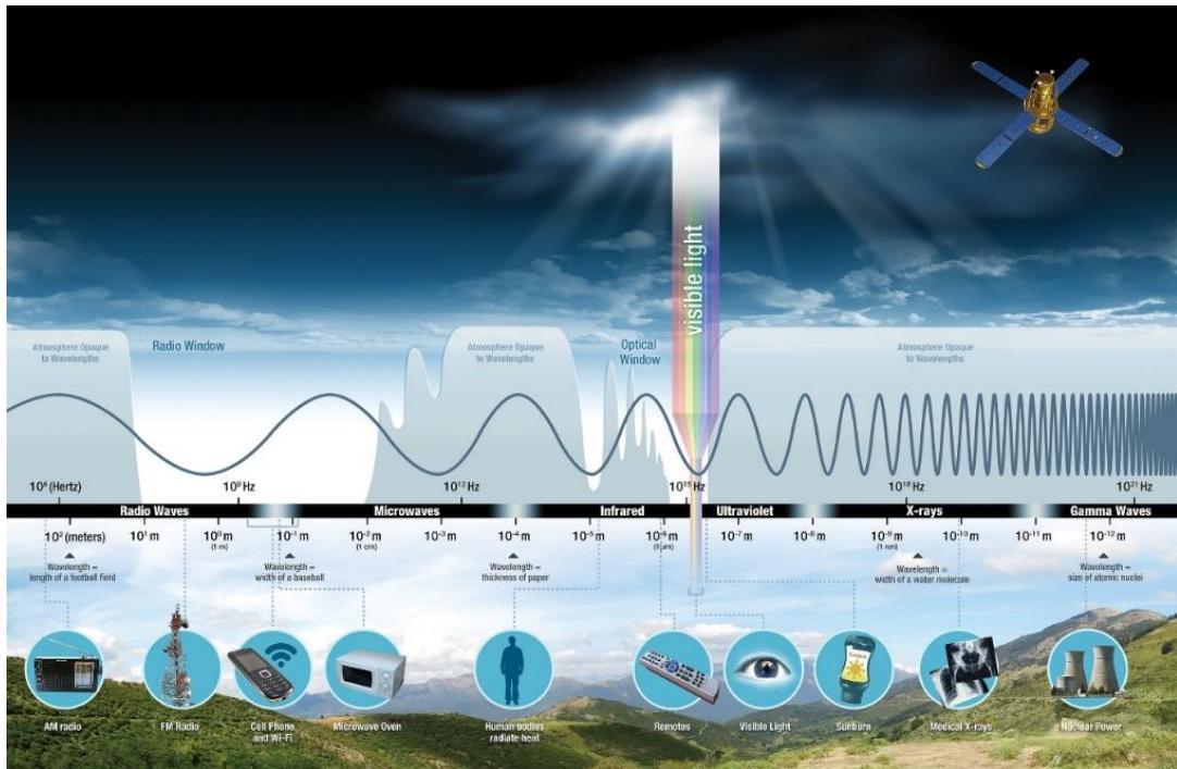
Obrázek 3 – atmosférická okna a elektromagnetické spektrum (science.nasa.gov).
