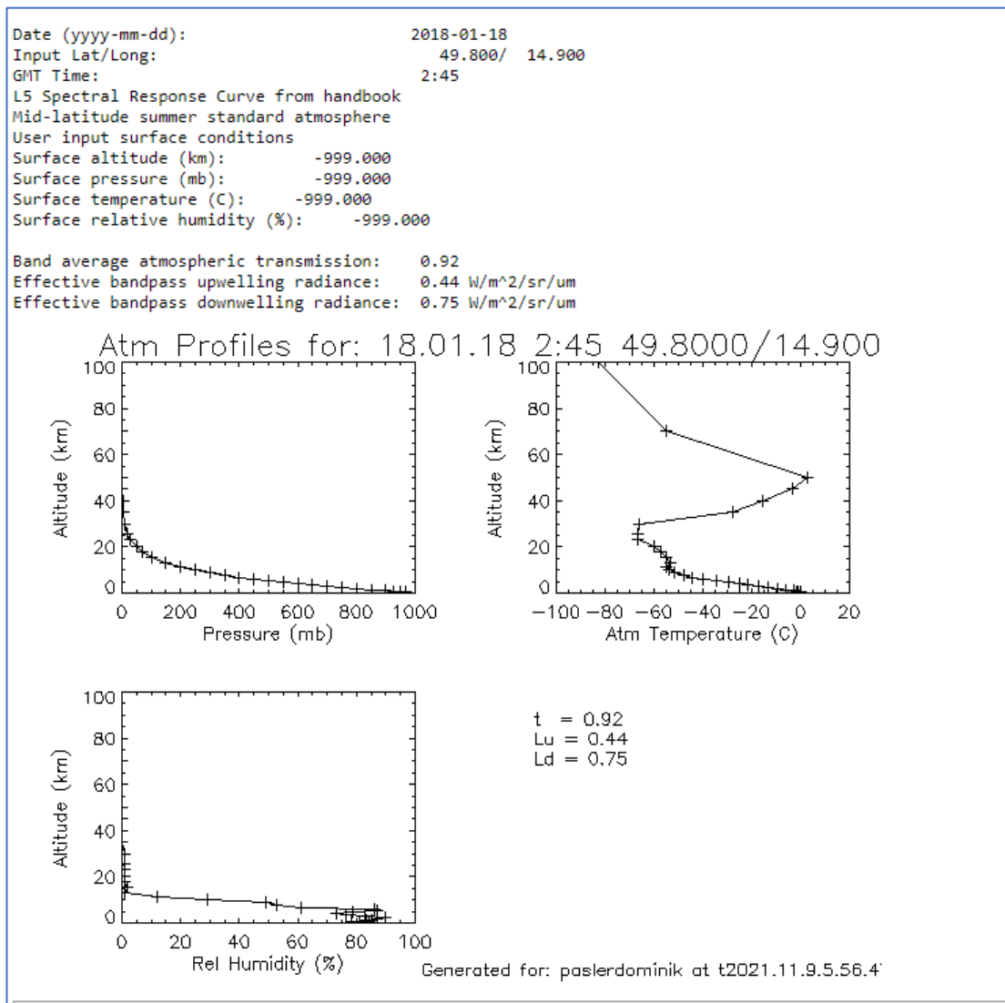
Obrázek 10 – výsledný profil atmosféry.
