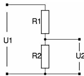
Obrázok č. 29: Napät'ový delič. [45]
