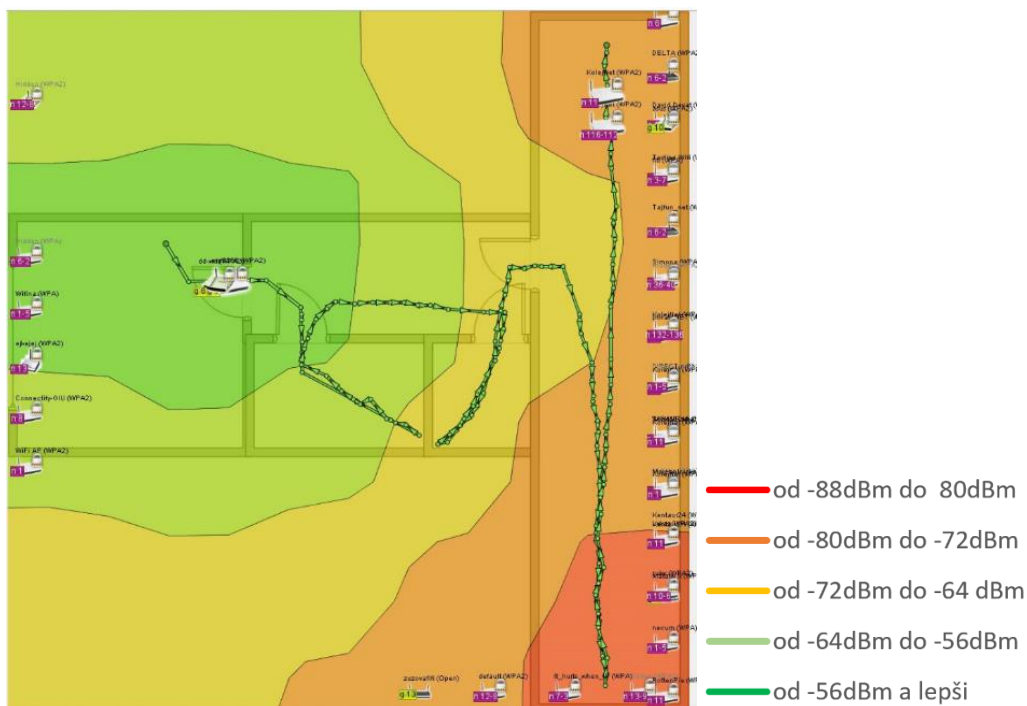
Obrázok č. 56: Meranie kvality Wi-Fi signálu pomocou programu Ekahau Heatmapper.
