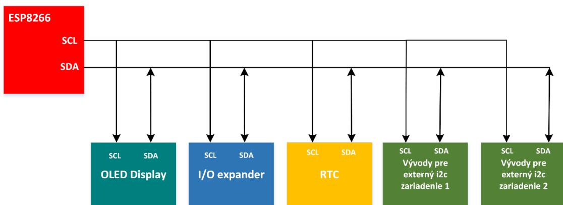
Obrázok č. 28: Bloková schéma zapojenia I2C zbernice s komponentami.
