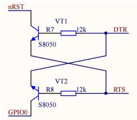
Obrázok č. 31: Schéma automatického reštartovania modulu ESP8266. [47]
