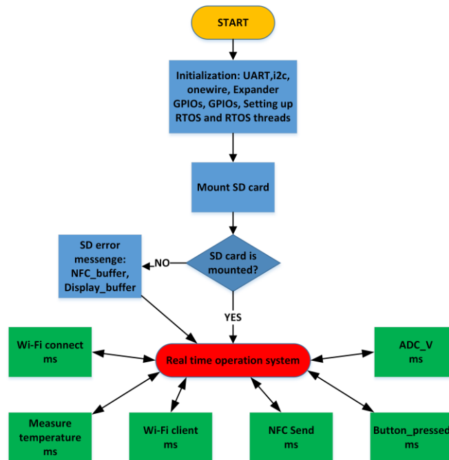
Obrázok č. 41: Vývojový diagram pre znázornenie funkčnosti RTOS v ESP8266.
