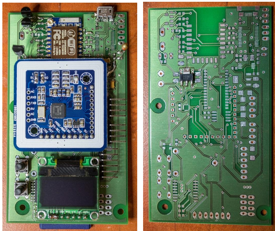
Obrázok č. 38: Výsledný oživovaný DPS a samotný DPS bez komponentov.
