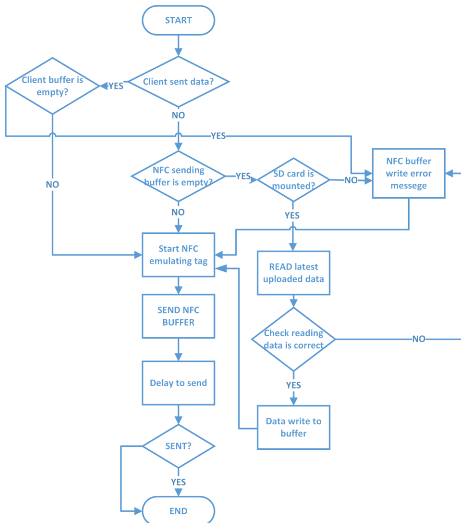
Obrázok č. 44: Vývojový diagram vlákna pre obsluhu NFC modulu.
