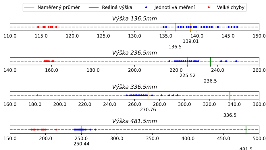
Obr. 2.2: Černý objekt (350x500mm)
