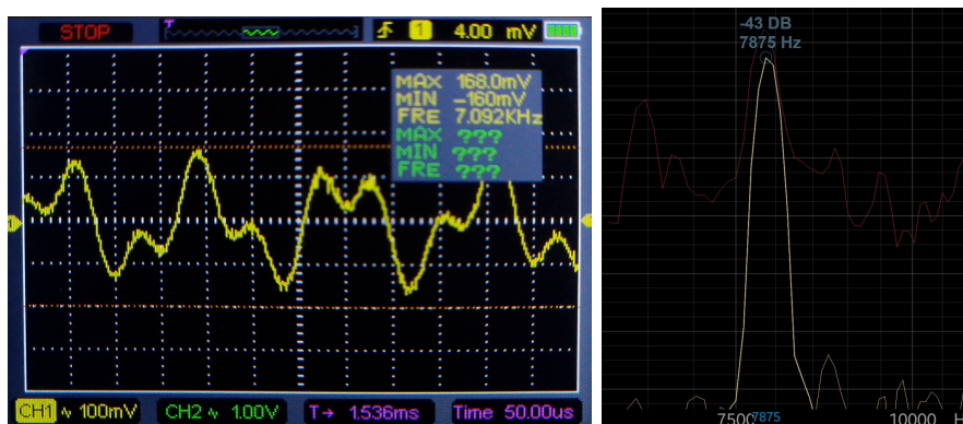
(a) Sinusová vlna–osciloskop (b) Sinusová vlna–Spectroid
