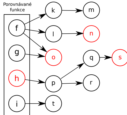
Obrázek 2.2: Příklad grafu volání, který zobrazuje porovnávané a sémanticky různé funkce. V obdélníku jsou znázorněny funkce, které jsou porovnávány. Hrany směřují z funkcí do funkcí jimi volaných. Červeně jsou označeny funkce, ve kterých je nalezen sémantický rozdíl.
