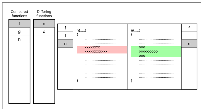
Obrázek 4.2: Prvotní návrh prohlížeče výsledků
