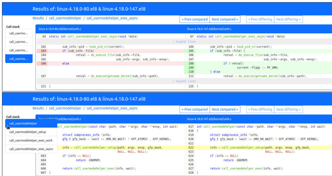
Obrázek 5.4: Snímky výsledného řešení zobrazení nalezeného rozdílu. Na horním snímku je zachyceno zobrazení zdrojového kódu funkce při výběru funkce s nalezeným sémantickým rozdílem ze zásobníku volání. Na dolním snímku je zachyceno zobrazení při výběru volající funkce (v tomto případě porovnávané funkce). Vytvořené řešení má na obrazovkách s nižším rozlišením zmenšený zásobník volání, který se zvětší při najetí kurzoru myši. Nezobrazené části kódu je možné zobrazit kliknutím na „Expand lines“. Jedná se o zobrazení stejného rozdílu, který byl zobrazen na Výpisu 2.1.
