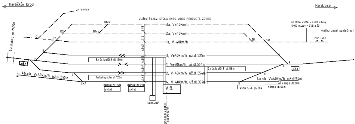
Obr. 1 Dopravní schéma žst. Ždírec nad Doubravou – stávající stav
