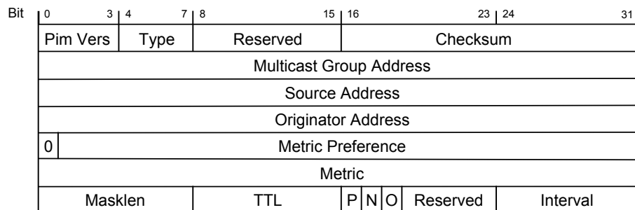
Obrázek 2.5: Formát PIM State Refresh zprávy.
