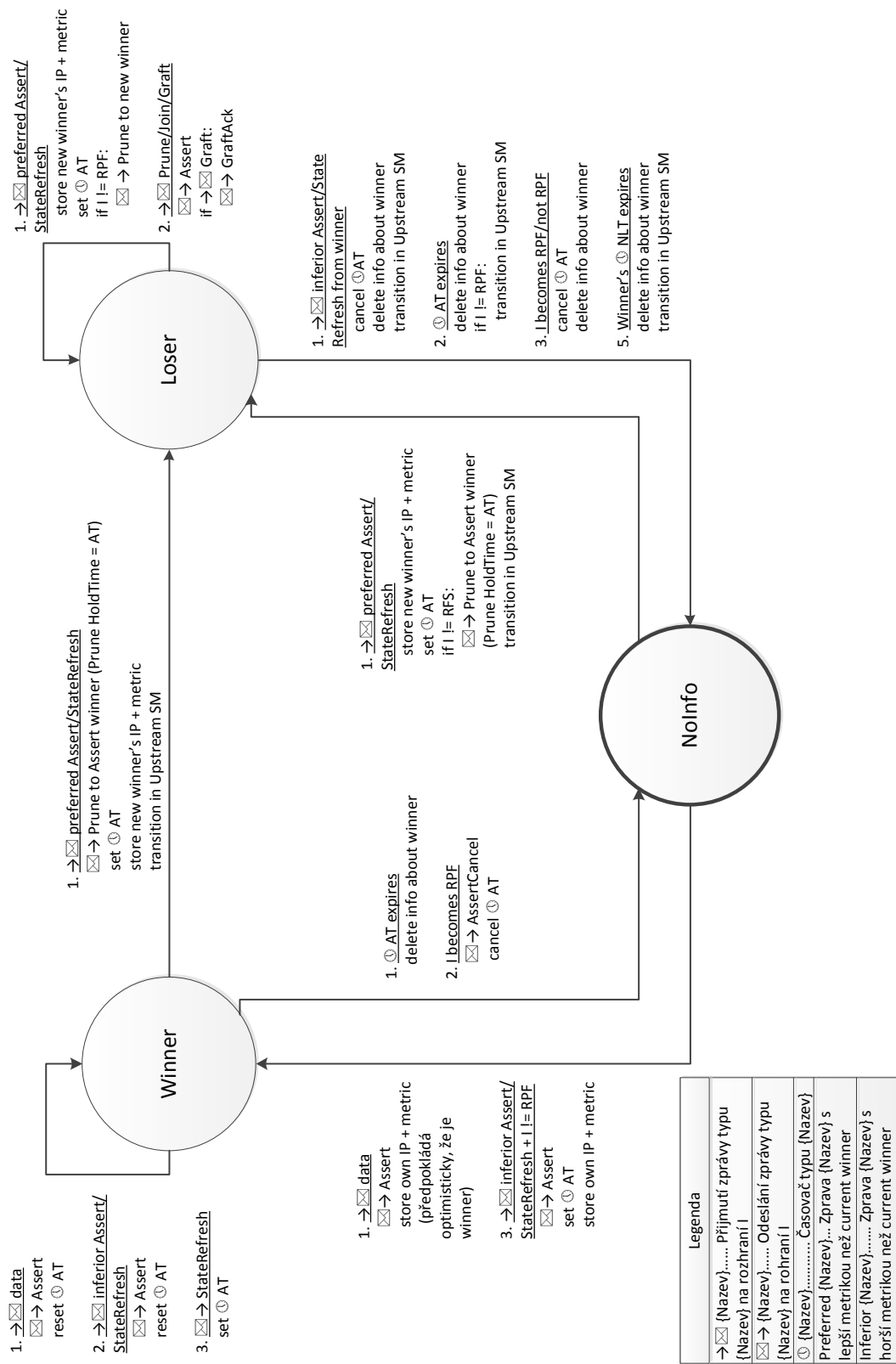
Obrázek 2.10: Assert Message (S,G,I) State Machine.
