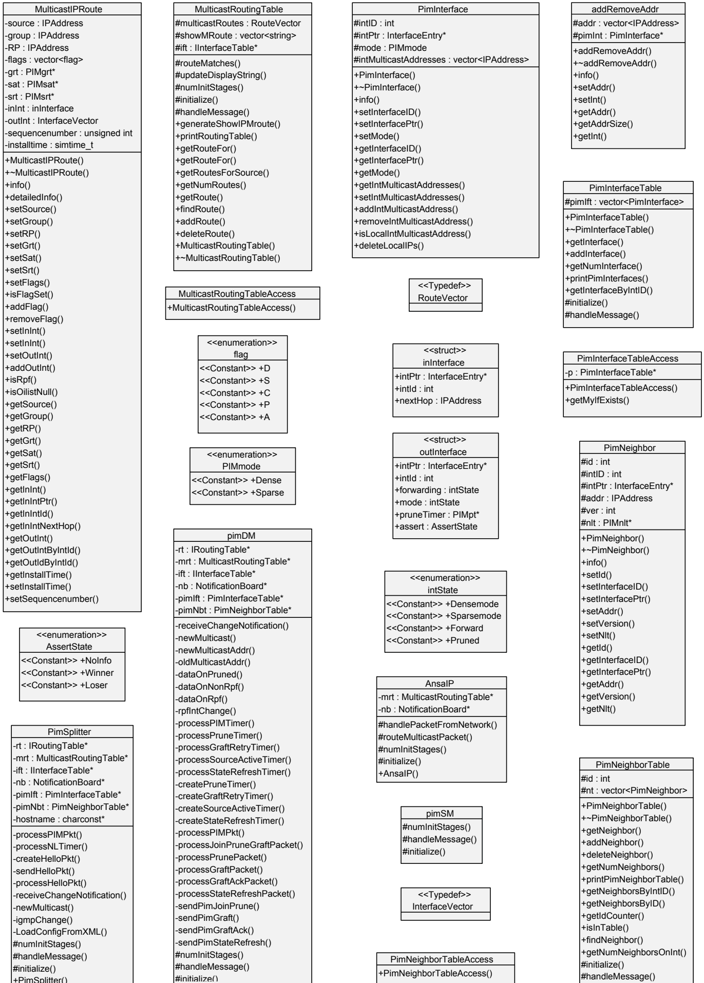
Obrázek C.1: Diagram tříd, které vznikli v rámci této práce.
