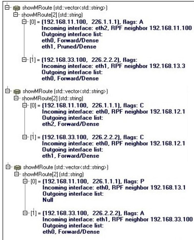
Obrázek 7.8: Multicastové směrovací tabulky směrovačů (shora) R1, R2 a R3 ze simulace (krok 4).
