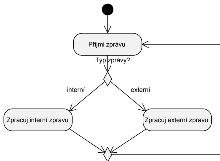
Obrázek 4.3: Základní diagram aktivity pro PIM-DM modul
