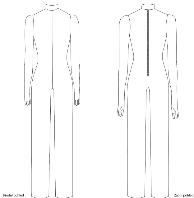
Obrázek 21: Technický náčrt overalu [21]
