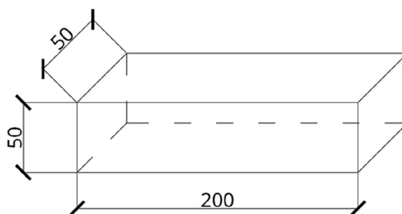
Obr. 30 Rozměry zkušebního tělesa
