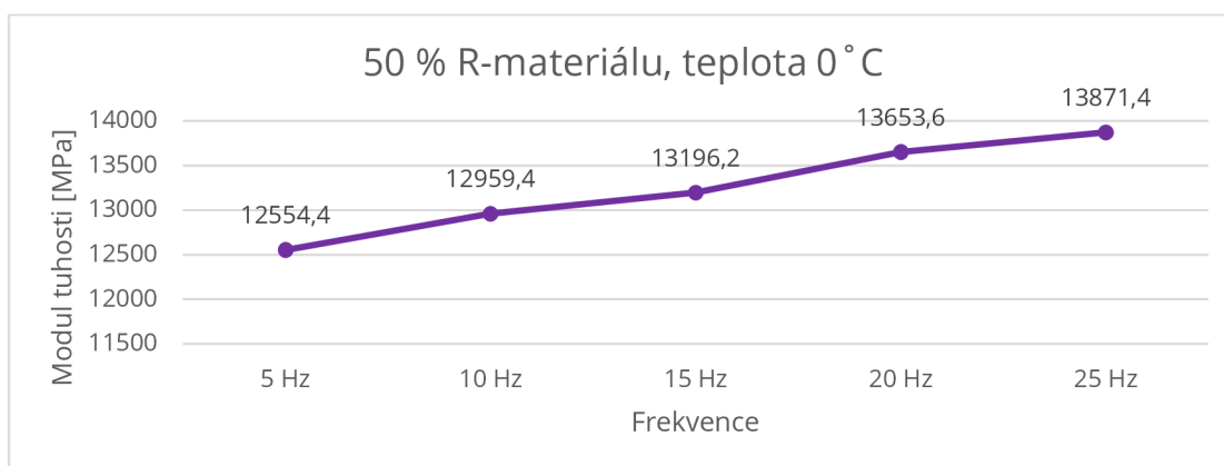
Graf 10 – Závislost modulu tuhosti na frekvenci, směs s 50 % R-materiálu při teplotě 0 °C
