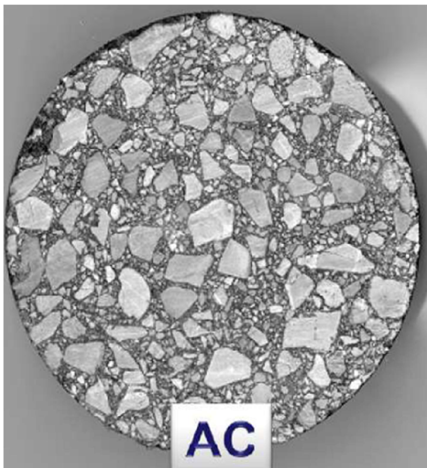
Obr. 6 Asfaltový beton - zkušební těleso [10]
