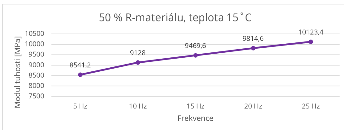
Graf 14 – Závislost modulu tuhosti na frekvenci, směs s 50 % R-materiálu při teplotě 15 °C
