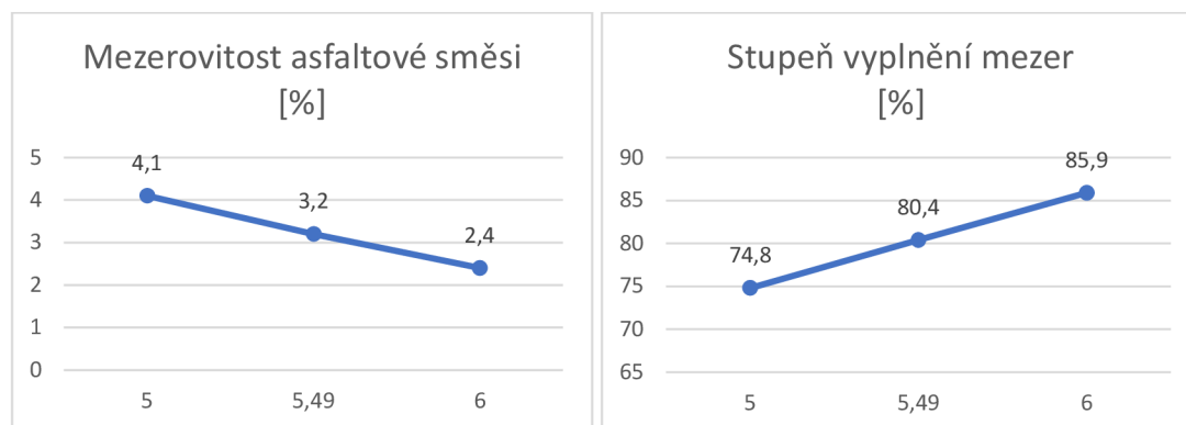
Graf 4: Mezerovitost asf. směsi
