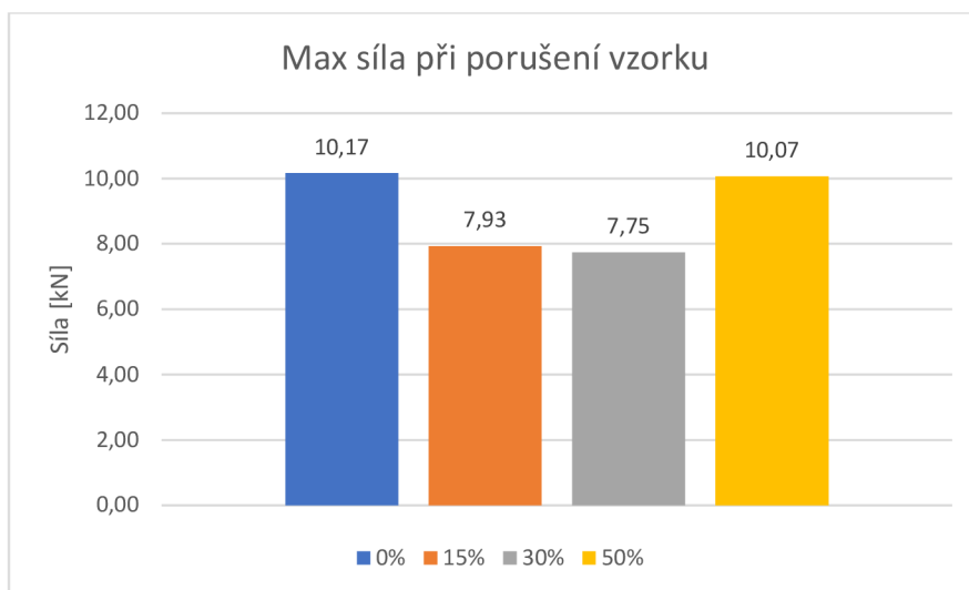
Graf 22: Zobrazení maximální síly porušení vzorku
