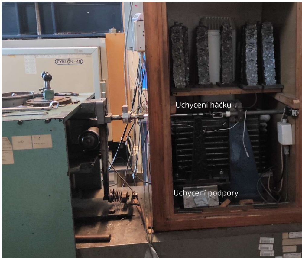
Obr. 27 Uchycení vzorku do temperovaného zařízení
