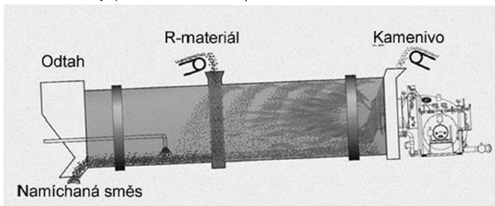
Obr. 16 Schéma kontinuální obalovny se systémem přidávání R-materiálu souběžně s proudem horkého vzduchu [19]
