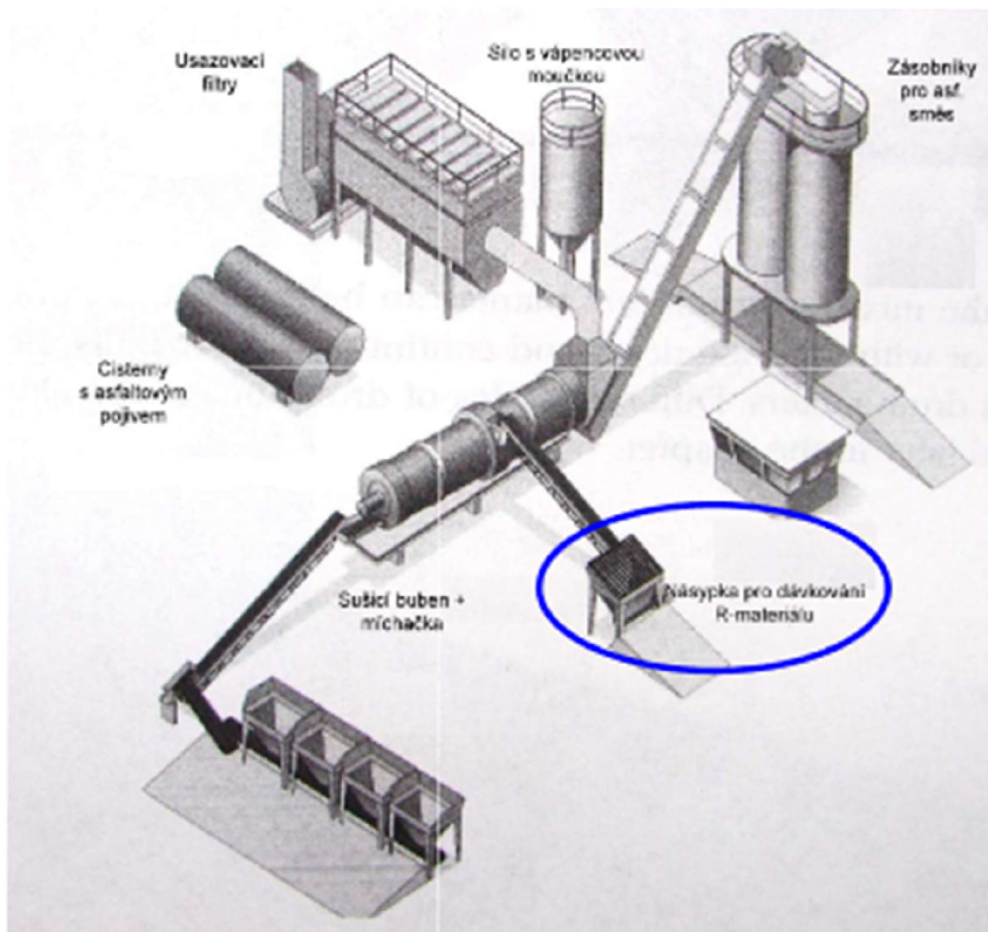
Obr. 15 Kontinuální obalovna Drum – mix [3]
