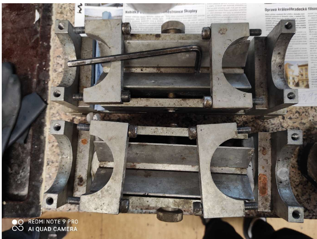
Obr. 29 Centrovací rám
