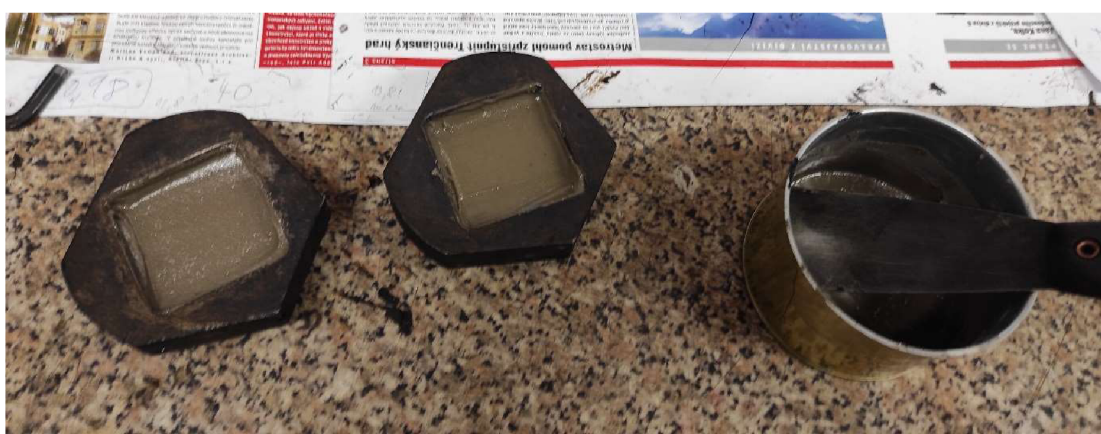
Obr. 23 Rozprostření lepidla do čelistí pro zkoušku posouzení nízkoteplotních vlastností
