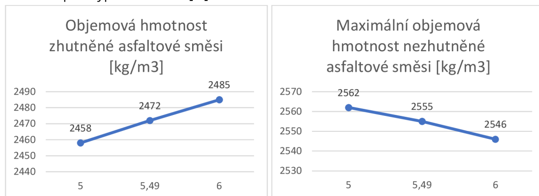
Graf 2,3: Objemové hmotnosti asfaltové směsi
