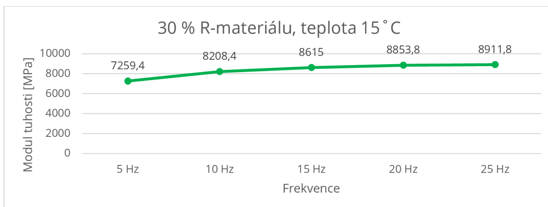
Graf 13 – Závislost modulu tuhosti na frekvenci, směs s 30 % R-materiálu při teplotě 15 °C
