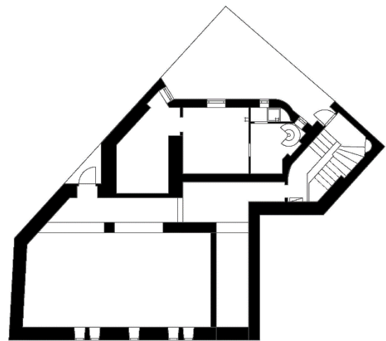
Obrázek 18: Generovaný půdorys
