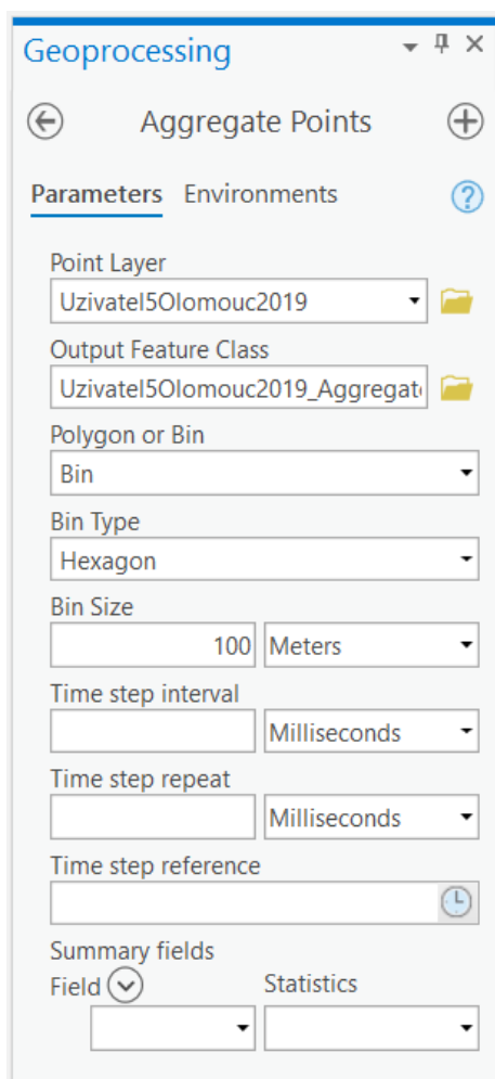
Obr. 4.1 – nastavenie nástroja Aggregate Points pri agregácii do hexagonálnej siete
