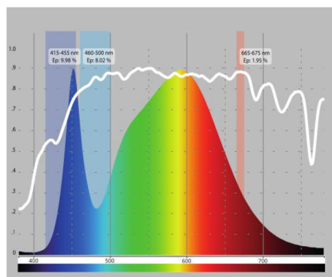
Obr. 2-15 Spektrální složení standardní LED [23]
