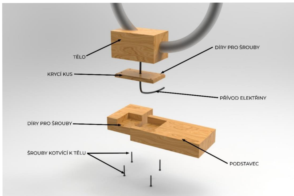
Obr. 6-6 Složení lampy
