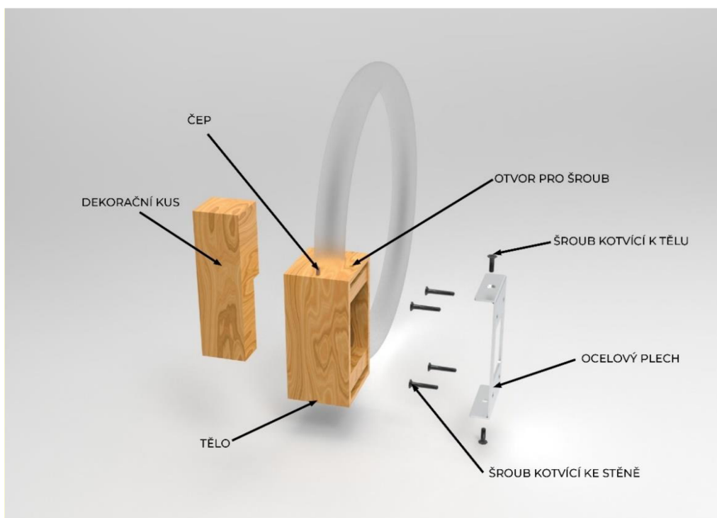
Obr. 6-9 Vnitřní mechanismy a komponenty nástěnného kusu
