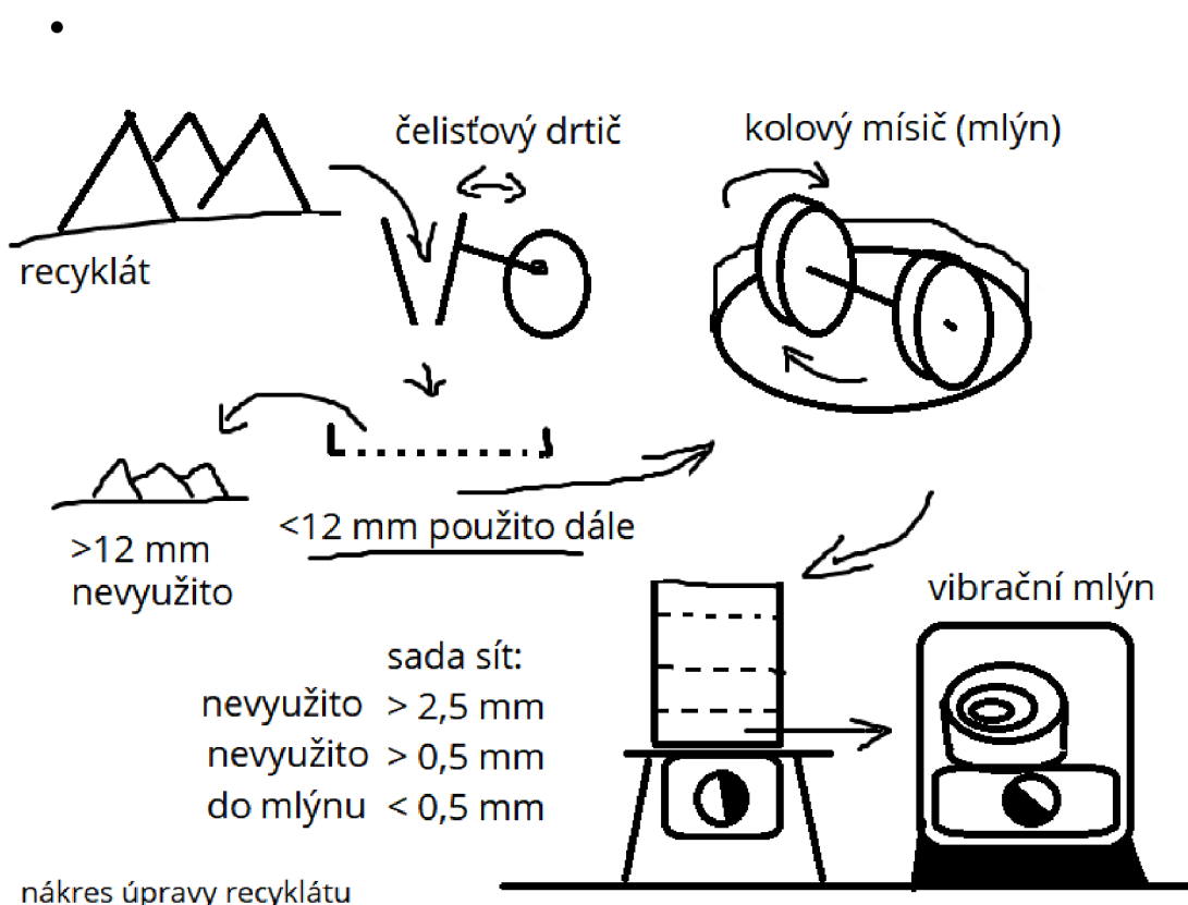
Obrázek 38: Nákres postupu při úpravě recyklátu - vlastní nákres
