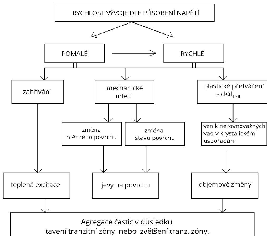
Vývojový diagram změn relaxačních procesů [Boldyrev 1986] - přeložil LuboOpat 19'
