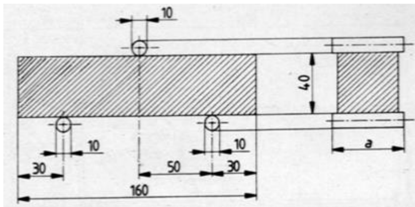
Obrázek 32: Provádění zkoušky v tahu za ohybu na trámečkách [54]
