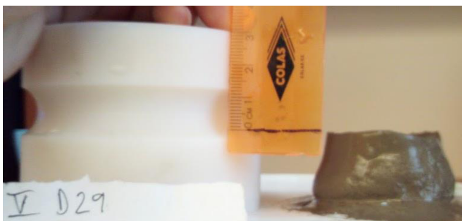
Obrázek 54: Reometrické vlastnosti - sednutí kužílku - D29
