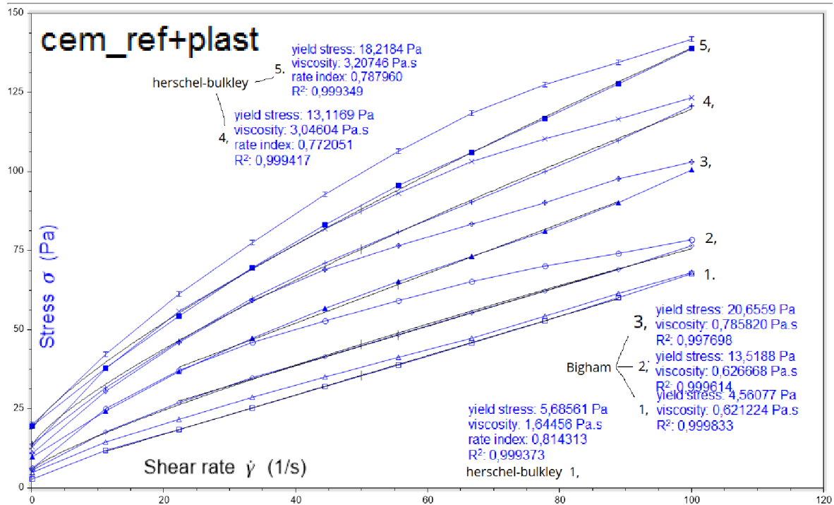
Obrázek 51: Měření reometrických vlastností - cem_ref
