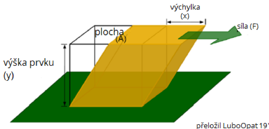
Obrázek 20: Obrázek pro odvození rovnice tečného napětí [41]
