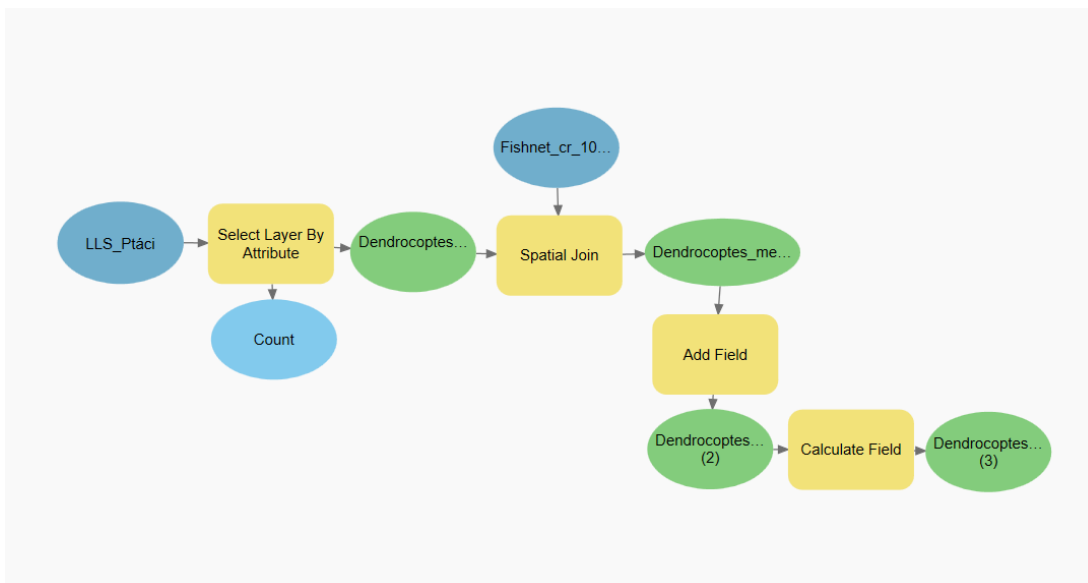
Obr. 8: Model vytvořený pomocí funkce ModelBuilder v ArcGIS Pro
