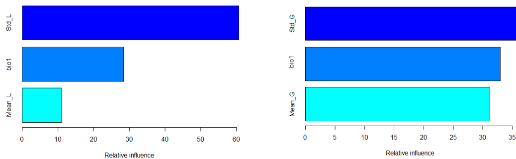
Obr. 17: Rozdíl v důležitosti sledovaných proměnných v případě použití dat LLS (vlevo) a GEDI (vpravo) u křivky obecné
