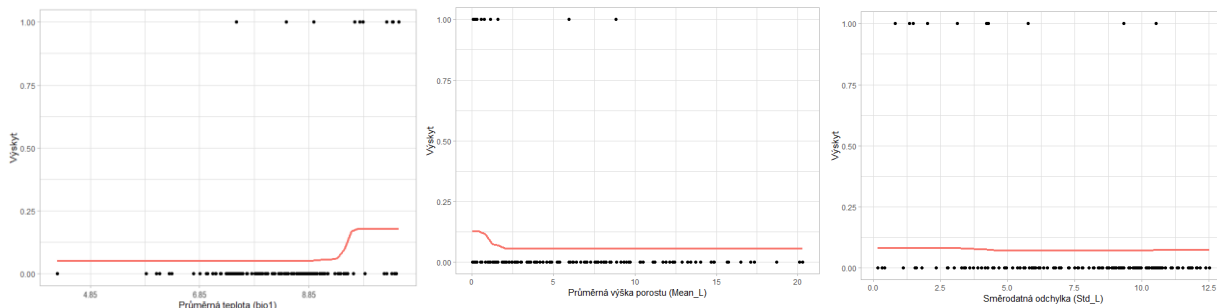
Příloha 5: Vliv proměnných na výskyt strakapouda jižního z leteckého laserového skenování.
