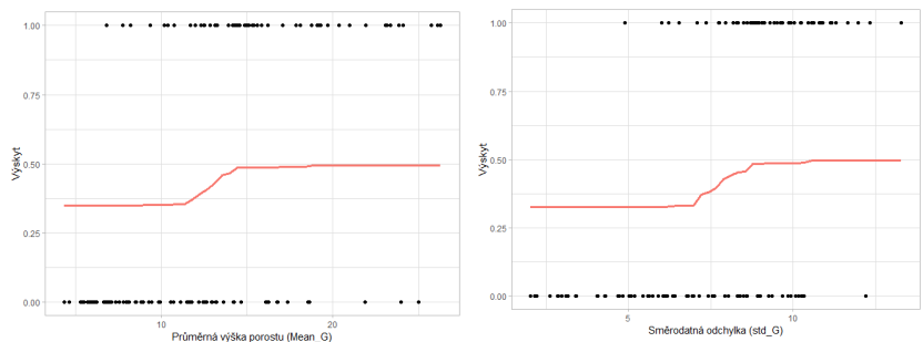
Příloha 31: Vliv proměnných na výskyt krivky obecné z mise GEDI.
