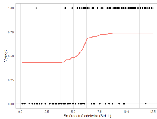
Obr. 13: Vliv směrodatné odchylky průměrné výšky vegetace z dat leteckého laserového skenování na pravděpodobnost výskytu sýkory uhelníčka
