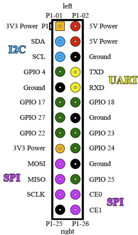
Obr. 2.2: Rozhraní GPIO.
