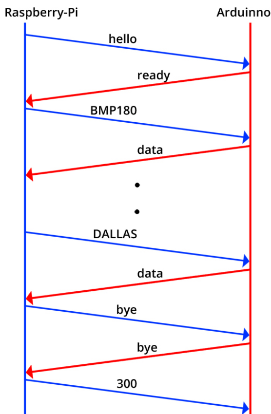
Obr. 3.3: Schéma komunikace mezi Raspberry Pi a Arduinem.
