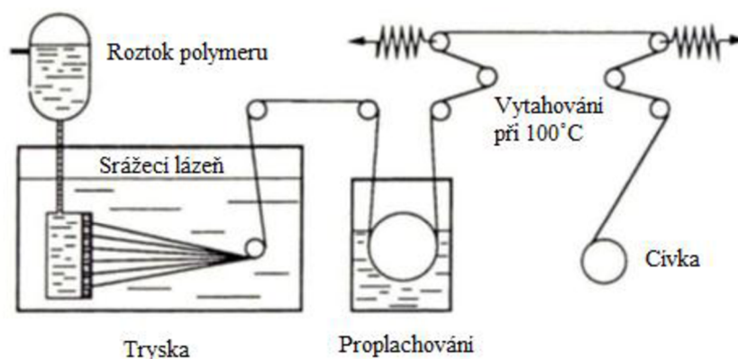
Obr. 26 Schéma spřádání [20].
