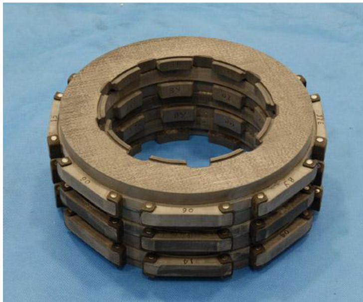
Obr. 34 Brzdové disky z letounu Boeing 757 [39].
