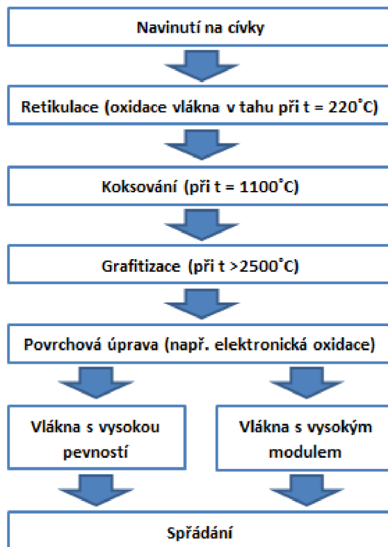
Obr. 25 Modelové schéma výroby PAN vláken.
