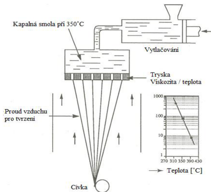
Obr. 28 Schéma spřádání [20].
