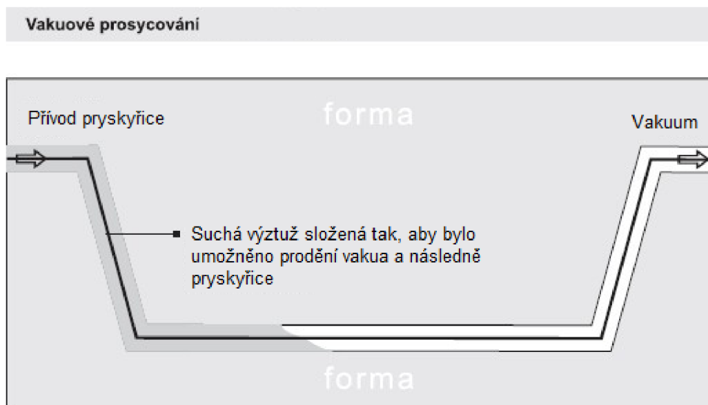
Obr. 9 Schéma vakuového prosycování [6].
