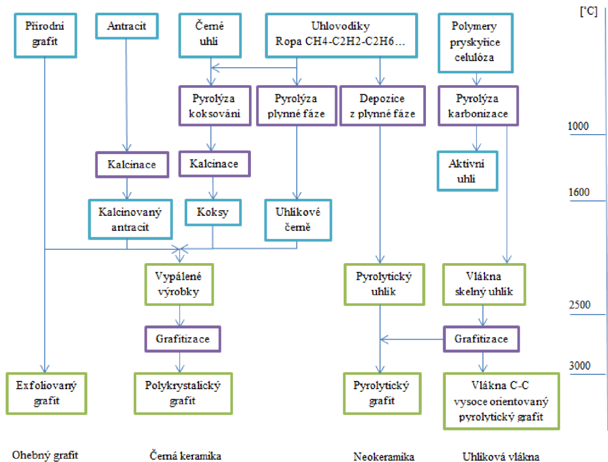
Obr. 18 Způsoby získávání uhlíkových materiálů [20].
