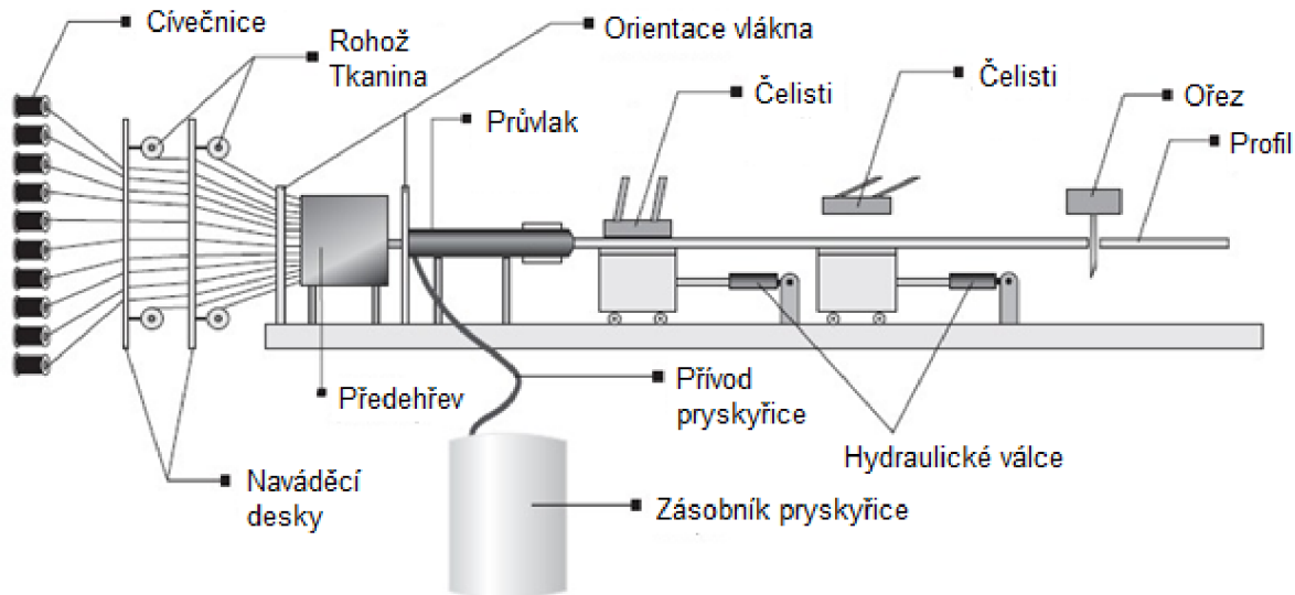
Obr. 10 Schéma tažení[6].
