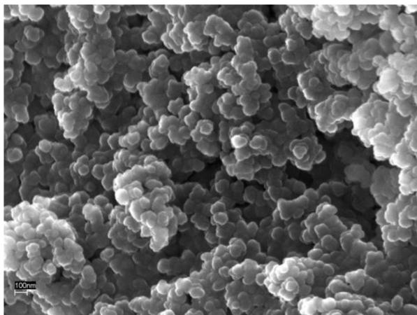
Obr. 22 Uhlíkový aerogel [28].
