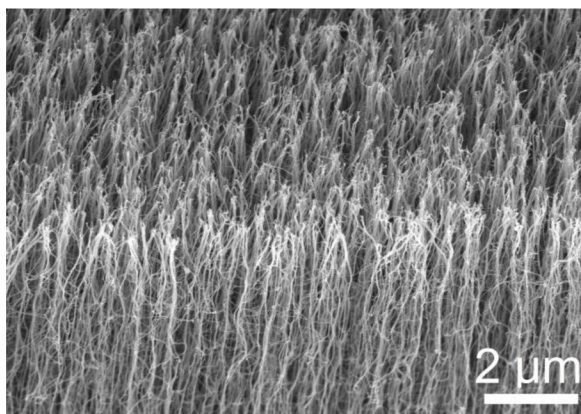
Obr. 23 Uhlíkové nanotrubičky [30].
