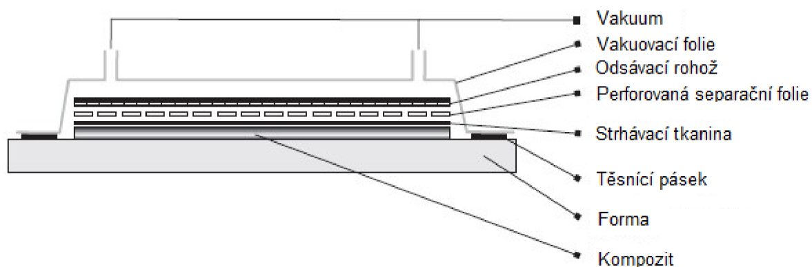
Obr. 7 Schéma lisování [6].
