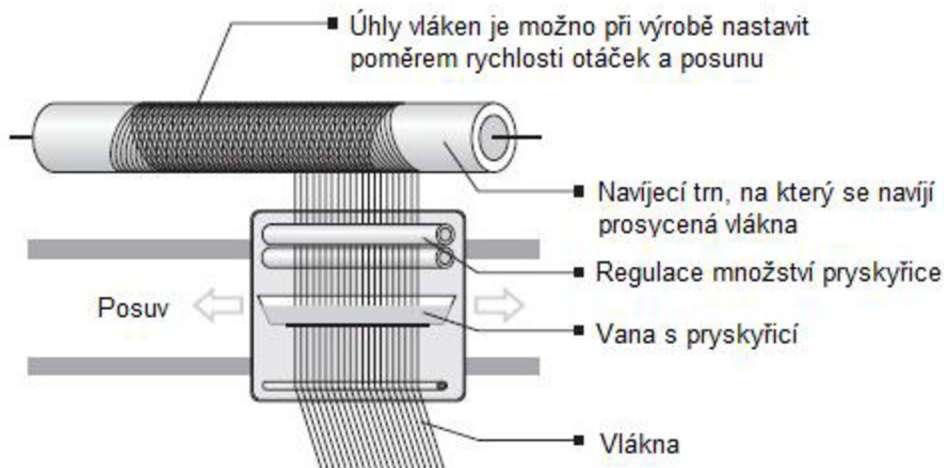
Obr. 11 Schéma navíjení [6].
