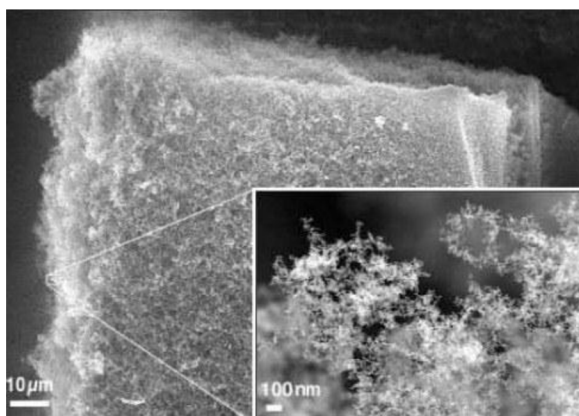
Obr. 22 Uhlíková nanopěna [29].
