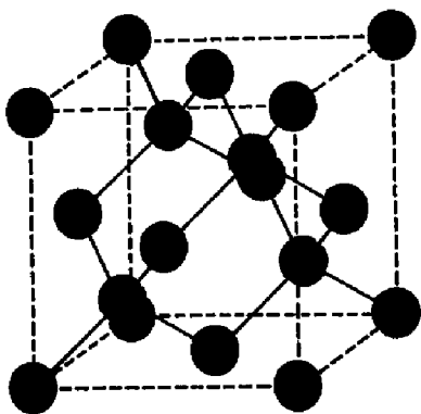
Obr. 14 Kubický diamant [17].
