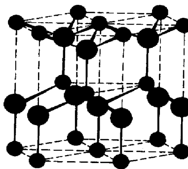
Obr. 15 Hexagonální diamant [17].
