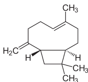
Obr. 6 – Strukturální vzorec \beta -karyofylenu
