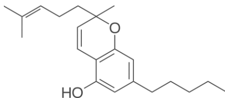
Obr. 4 – Strukturní vzorec CBC
