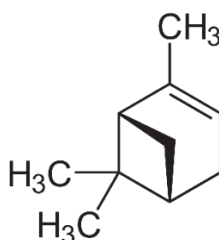
Obr. 6 – Strukturní vzorec pinenu
