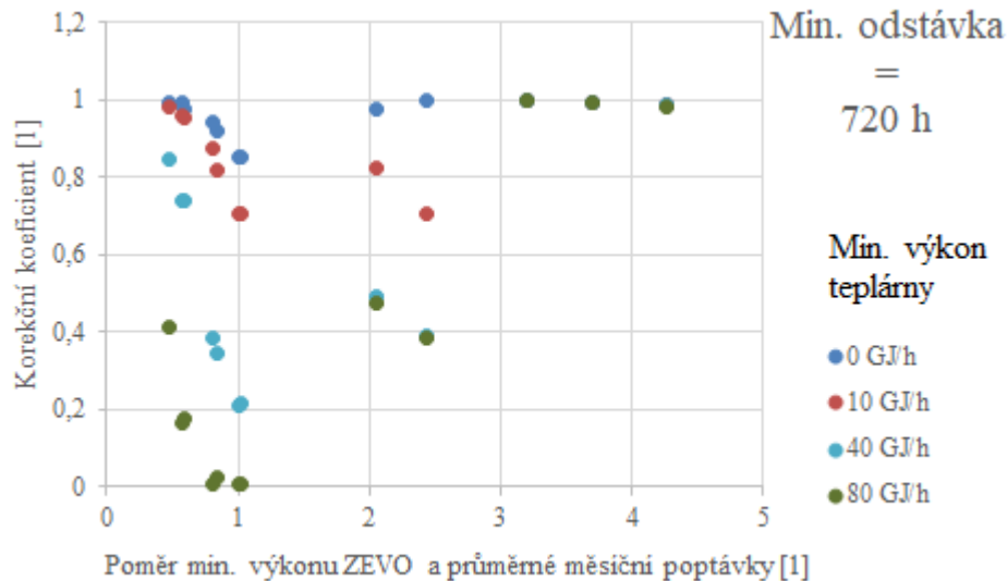
Obrázek 4.9: Korekční koeficienty při minimální době odstávky 720 hodin
