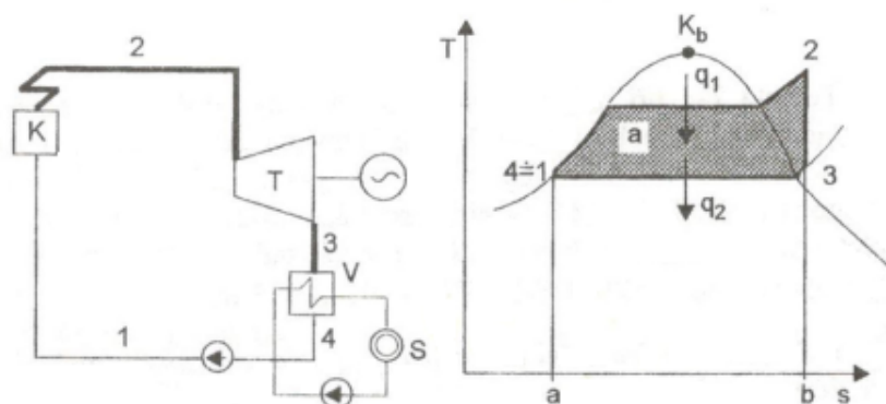
Obrázek 1.4: Schéma teplárny s kondenzační turbínou [15]
