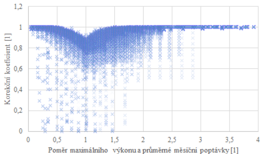
Obrázek 4.5: Závislost všech korekčních koeficientů na poměru max. výkonu a poptávky
