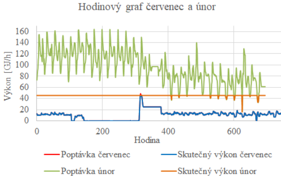
Obrázek 4.1: Skutečná a teoretická dodávka tepla za červenec a únor
