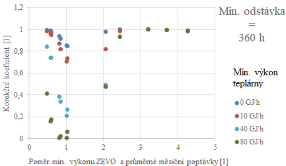
Obrázek 4.8: Korekční koeficienty při minimální době odstávky 360 hodin
