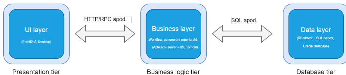
Obrázek 2.3: Ukázka rozložení layers mezi tiers – vrstvy – ve třívrstvé architektuře, inspirováno a doplněno [5]
