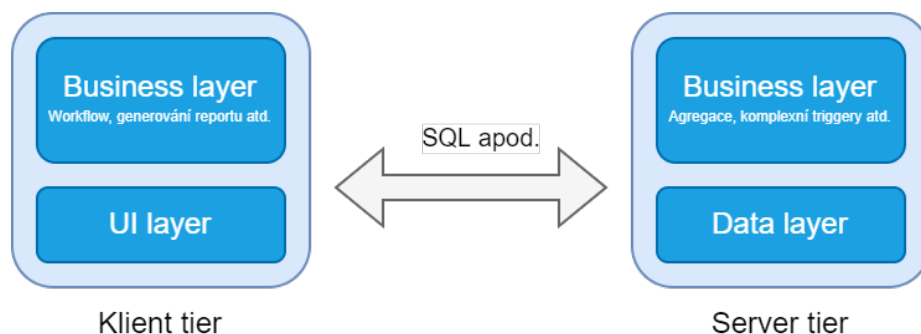
Obrázek 2.1: Ukázka rozložení layers mezi tiers – vrstvy – ve dvouvrstvé architektuře, inspirováno a doplněno [5]
