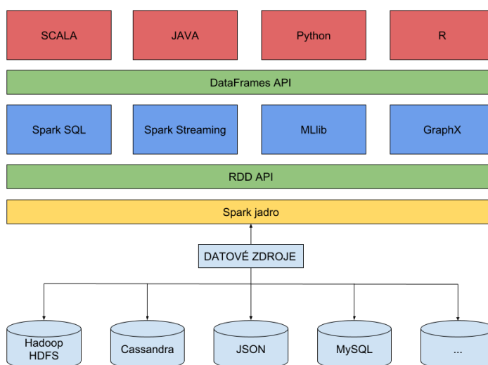
Obr. 2.1 Spark architektúra
