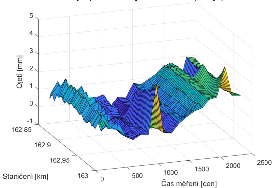
Graf ojetí po délce koleje v čase - úsek 1, kolej 1, SL
