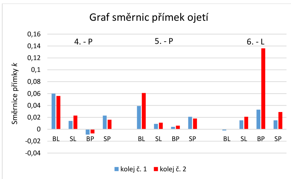
Obr. 9.8 – Graf směrnic přímků ojetí pro úseky č. 4, 5 a 6
