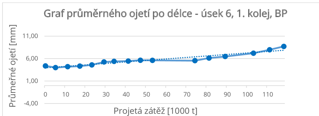
Obr. 9.63 – Graf průměrného ojetí – úsek 6, kolej č. 1, BP
