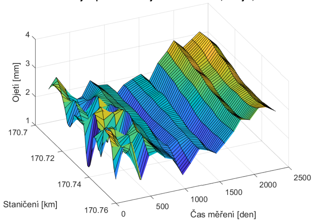
Graf ojetí po délce koleje v čase - úsek 3, kolej 2, SP
