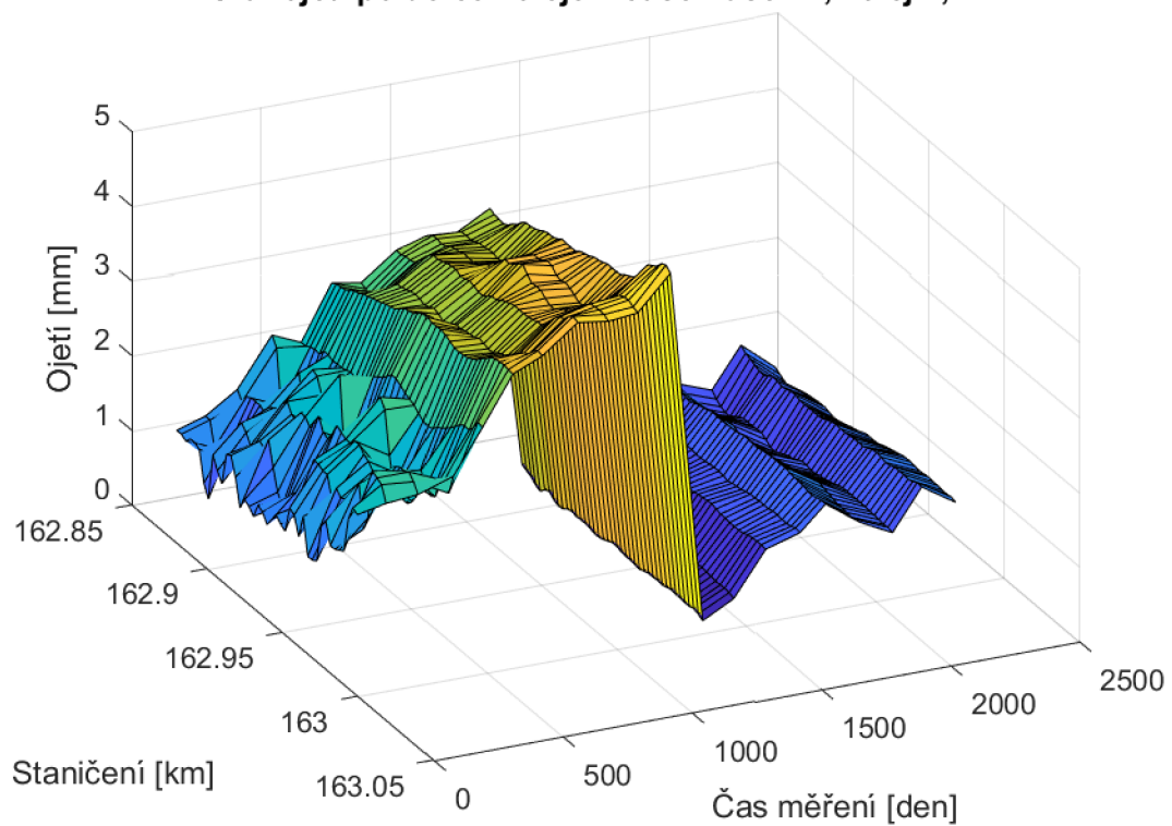
Graf ojetí po délce koleje v čase - úsek 1, kolej 2, BP
