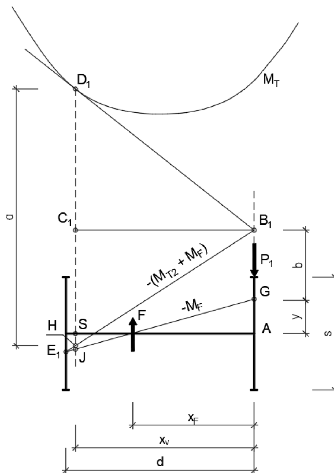
Obr. 6.7 – Grafická metoda pro vzpříčenou polohu s vnější silou F Informace byly získány z literatury [3] a [4].
