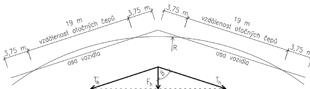
Obr. 7.3 – Rozklad síly
