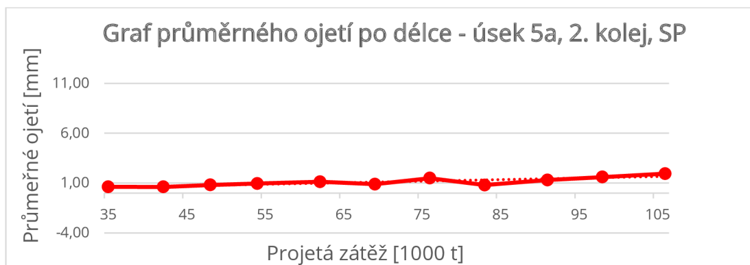
Obr. 9.56 – Graf průměrného ojetí – úsek 5a, kolej č. 2, SP
