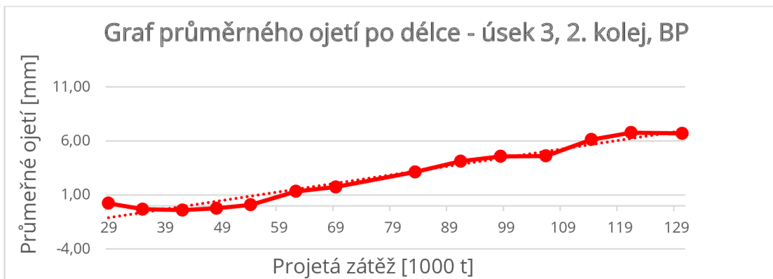
Obr. 9.39 - Graf průměrného ojetí - úsek 3, kolej č. 2, BP
