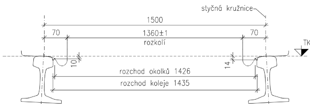
Obr. 5.2 – Příčný řez kolejí
