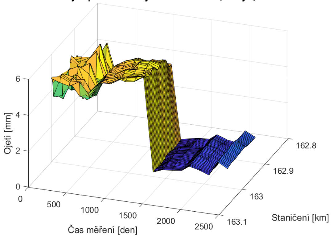
Graf ojetí po délce koleje v čase - úsek 1, kolej 2, SP
