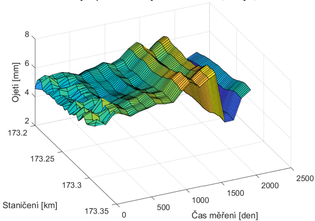
Graf ojetí po délce koleje v čase - úsek 4, kolej 2, SP
