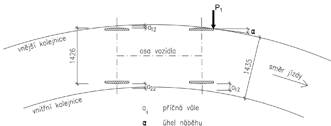
Obr. 5.1 – Zobrazení vodorovného řezu dvounápravovým podvozkem
