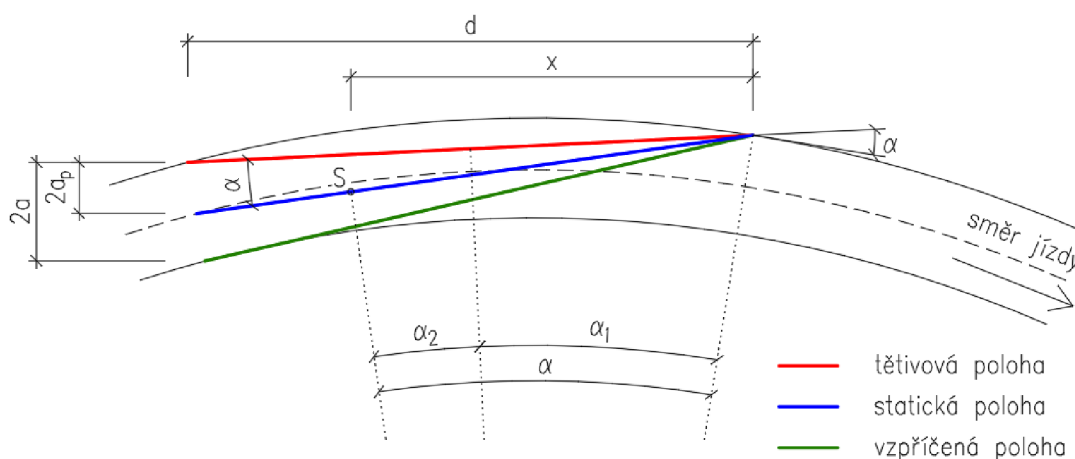
Obr. 5.3 – Polohy podvozku
