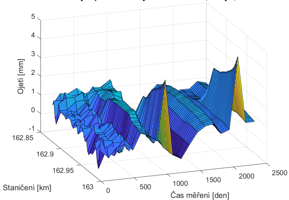
Graf ojetí po délce koleje v čase - úsek 1, kolej 1, SP
