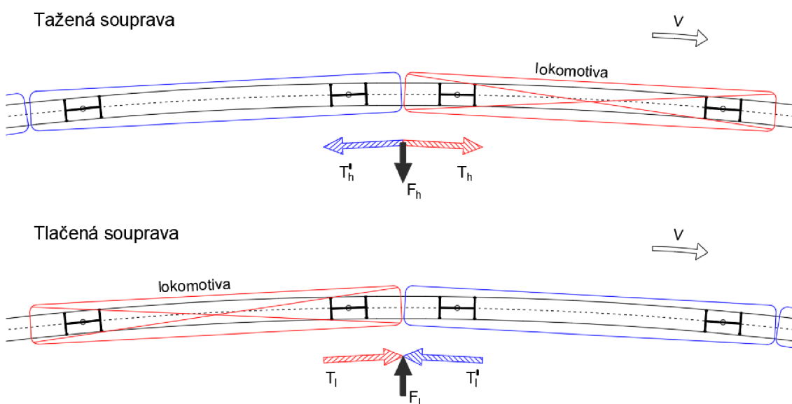
Obr. 7.2 – Silový rozdíl mezi taženou a tlačnou soupravou
