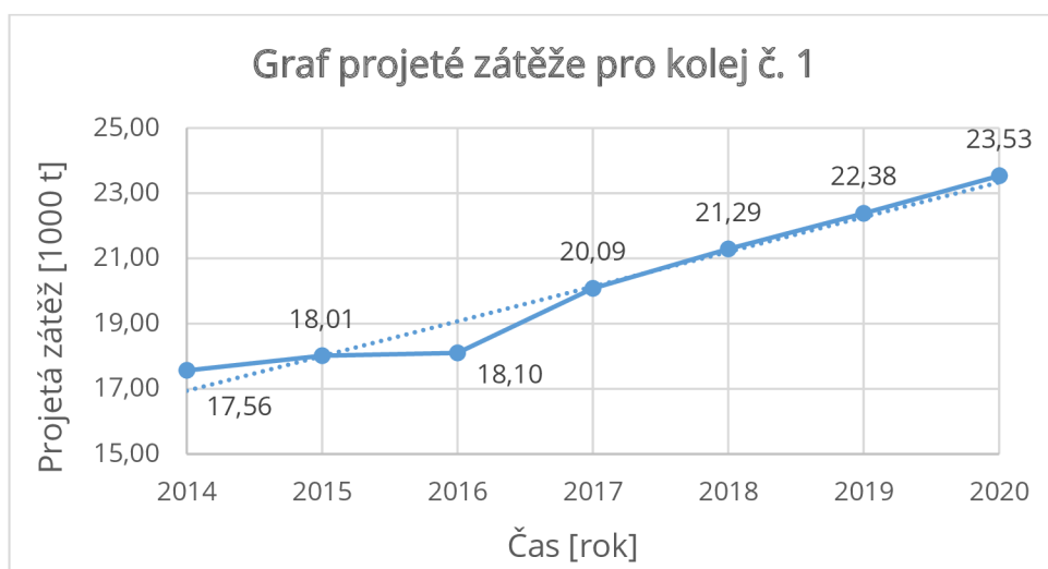
Obr. 9.4 – Graf projeté zátěže pro kolej č. 1
