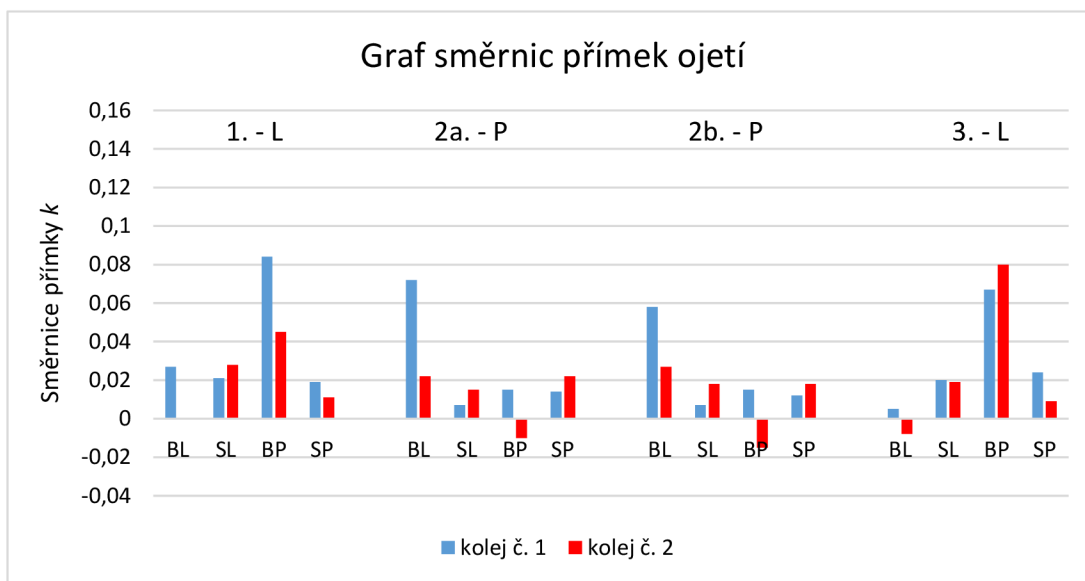
Obr. 9.7 – Graf směrnic přímků ojetí pro úseky č. 1, 2a, 2b a 3
