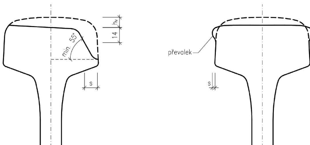
Obr. 8.1 – Příklad ojetí hlavy kolejnic
