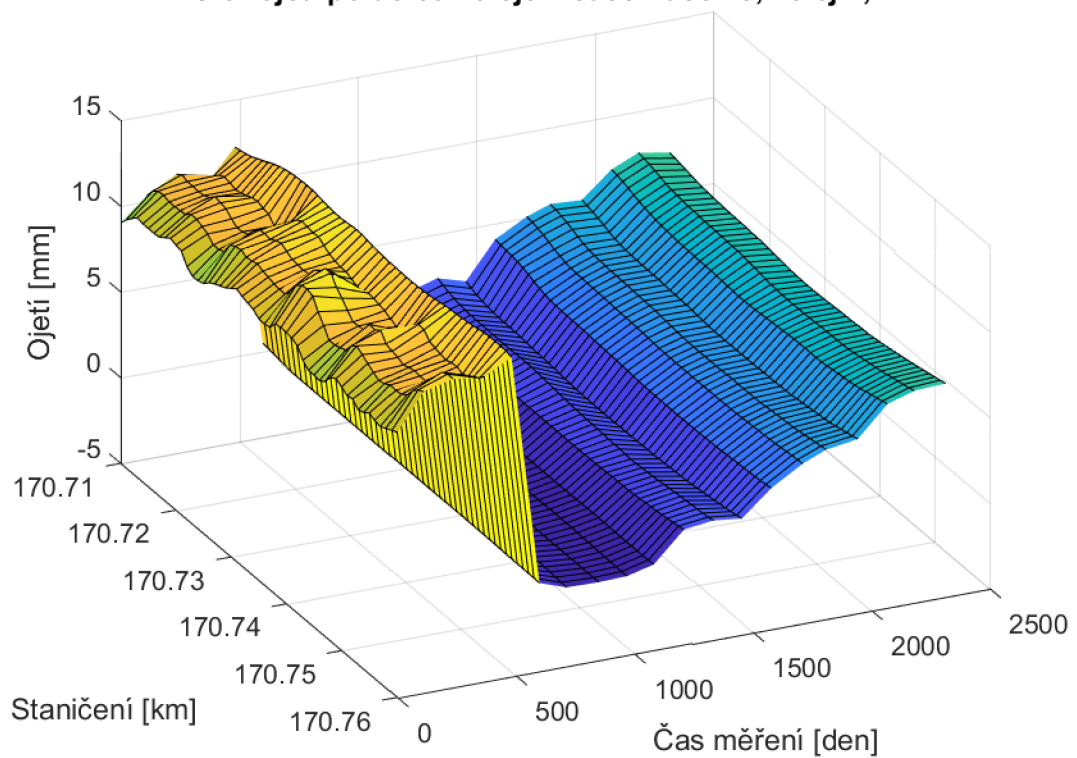
Graf ojetí po délce koleje v čase - úsek 3, kolej 2, BP
