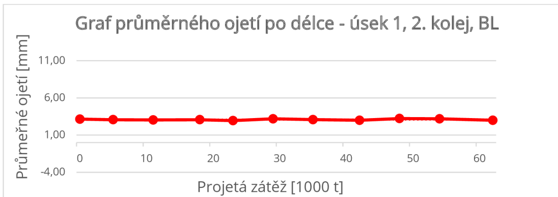
Obr. 9.13 - Graf průměrného ojetí - úsek 1, kolej č. 2, BL
