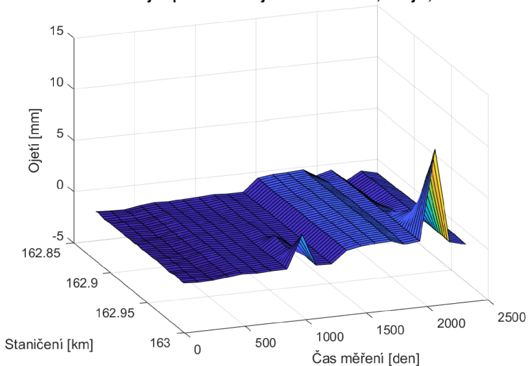
Graf ojetí po délce koleje v čase - úsek 1, kolej 1, BL
