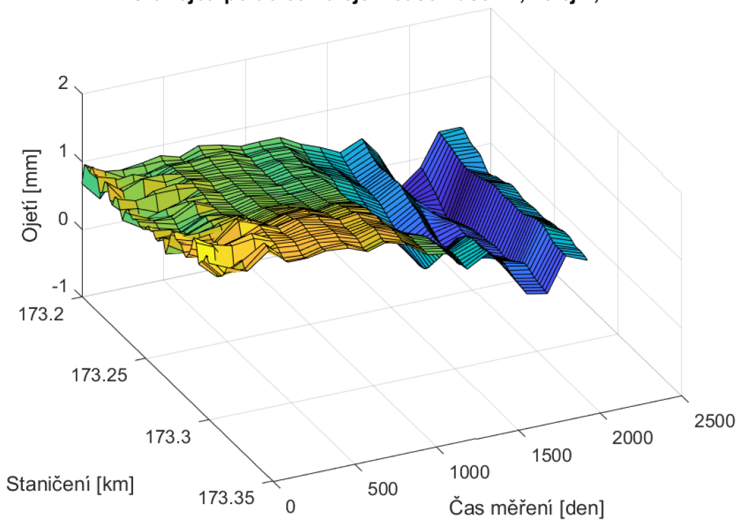
Graf ojetí po délce koleje v čase - úsek 4, kolej 2, BP
