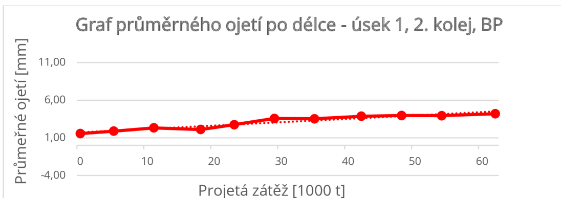
Obr. 9.15 - Graf průměrného ojetí - úsek 1, kolej č. 2, BP
