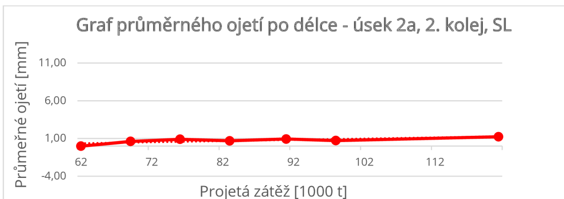
Obr. 9.22 - Graf průměrného ojetí - úsek 2a, kolej č. 2, SL
