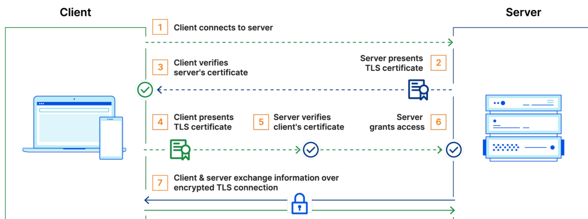
Obrázek 9 - mTLS (Cloudflare, 2024)
