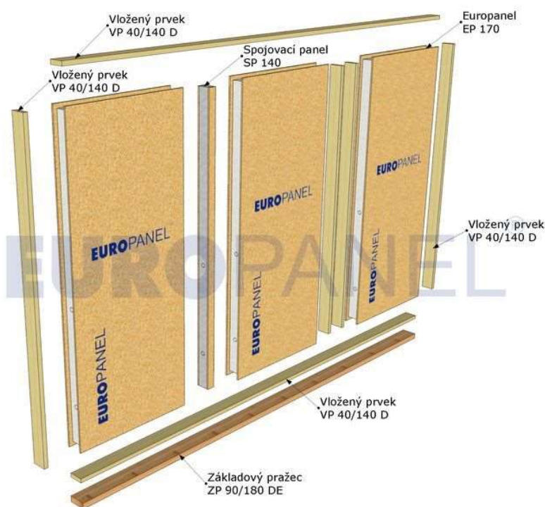
Obrázek 3. Stavební systém z europanelů (Europanel, 2017)
