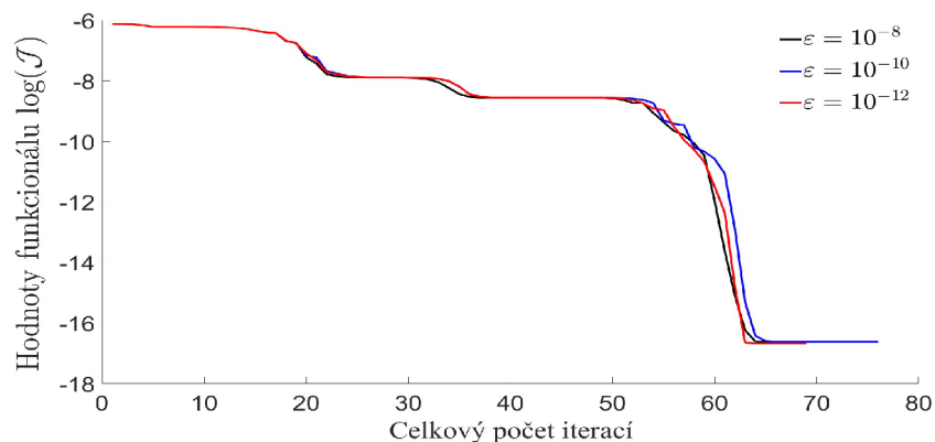
Obrázek 8: Hodnoty cenového funkcionálu \mathcal{J} během výpočtu pro \epsilon a 4 segmenty.
