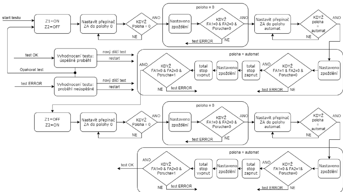
Obrázek 36 - Vývojový diagram testu výpadku bezpečnostním tlačítkem
