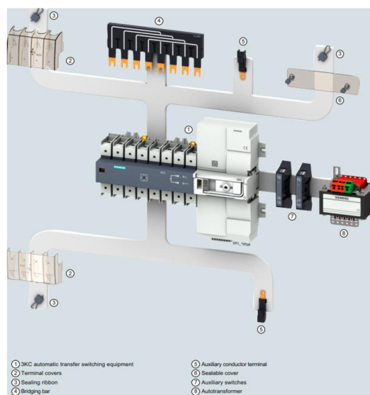
Obrázek 5 - Siemens 3KC6 záskokový automat s příslušenstvím [8]
